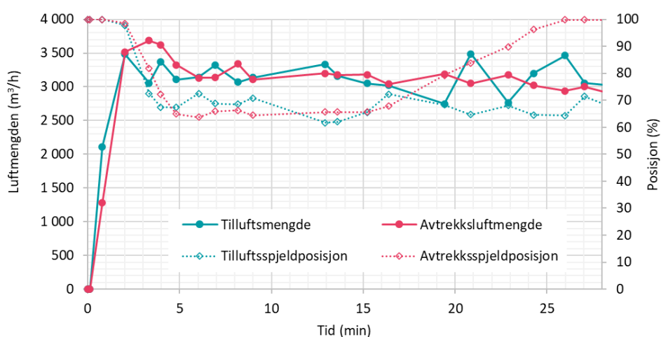
Figur 4-84: Luftmengder målt med SD anleggets sensorer og spjeldposisjoner i «resten av skolen» tilluft og avtrekk for test 13.
