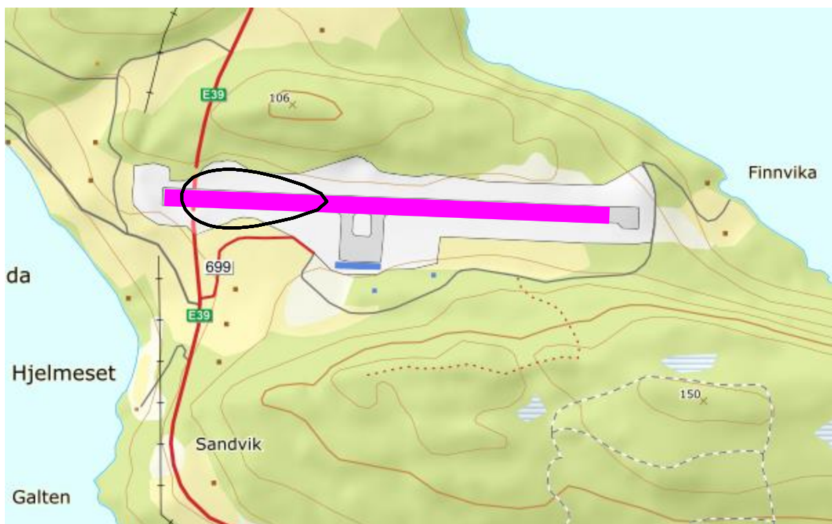
Figur 10-5. L_{\text{night}} for dagens situasjon (2017) i 5 dB trinn fra 50 dBA. Det er så lite trafikk på natt at bare koten for 50 dBA er definert. M 1:10 000.
