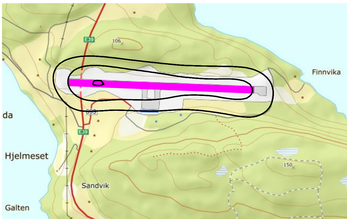
Figur 10-3. L_{den} for dagens situasjon (2017) i 5 dB trinn fra 50 dBA. M 1:10 000.
