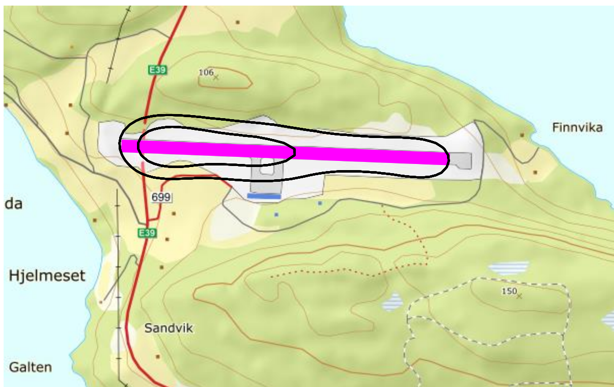
Figur 10-1. Kartleggingsgrenser for dagens situasjon (2017). L_{Aeq,24h} 51 og 54 dBA. M 1:10 000.
