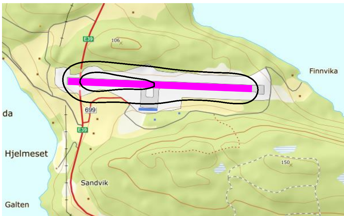
Figur 10-8. L_{Aeq,24h} for prognosesituasjonen (2028) i 5 dB trinn fra 50 dBA. M 1:10 000.
