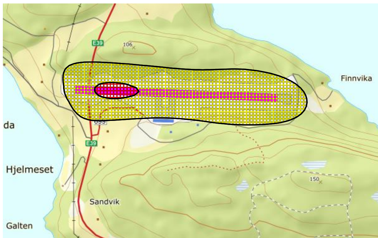
Figur 9-2. Rød og gul støysone for Sandane lufthamn, Anda, for prognosesituasjonen (2028). M 1:10 000.
