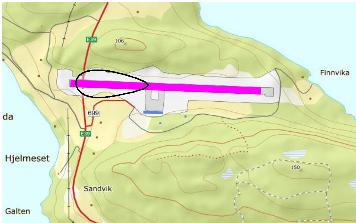
Figur 10-6. L_{\text{night}} for prognosesituasjonen (2028) i 5 dB trinn fra 50 dBA. Det er så lite trafikk på natt at bare koten for 50 dBA er definert. M 1:10 000.
