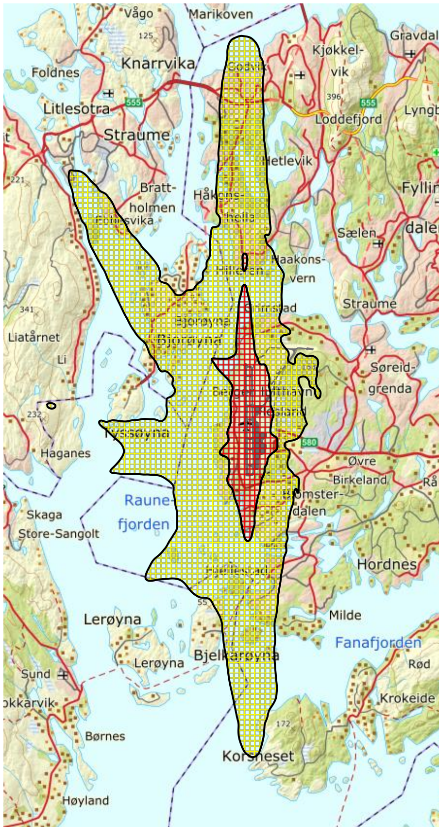
Figur 9-3. Rød og gul støysone for prognosesituasjon (2028), samlet trafikk. M 1:100 000.
