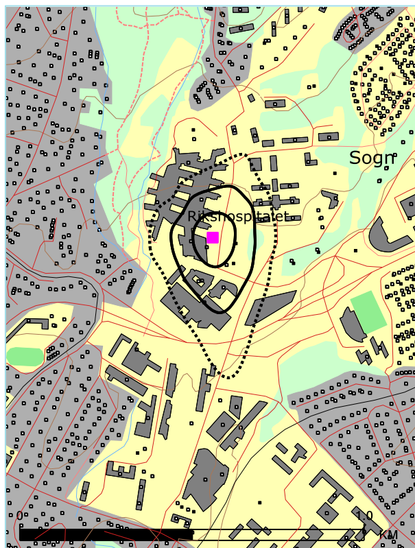
Figur 10-1. Kartleggingsgrenser i henhold til forurensningsforskriften. Kotene viser L_{Aeq,24h} 51 (stiplet), 54 og 61 dBA. Målestokk 1:10 000.
