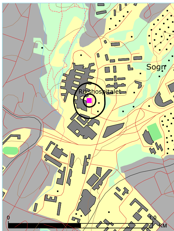
Figur 9-2. L_{5AS} 80 og 90 dBA for dagens situasjon. M 1:15 000.
