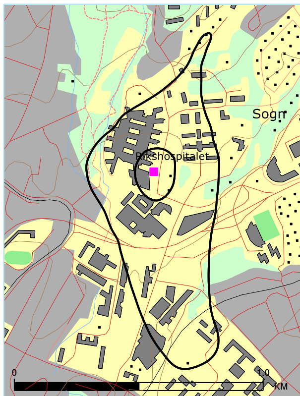
Figur 9-1. L_{den} 52 og 62 dBA for dagens situasjon. M 1:15 000.
