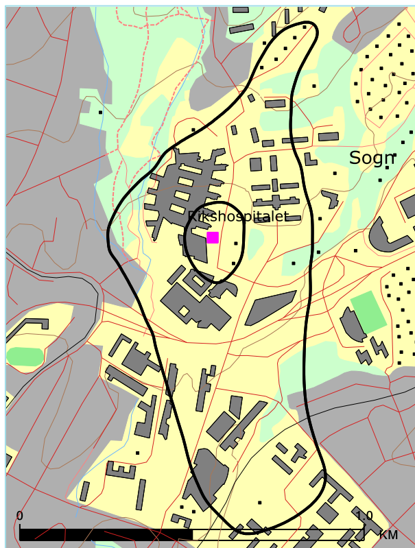
Figur 9-3. L_{den} 52 og 62 dBA for prognosesituasjonen. M 1:15 000.
