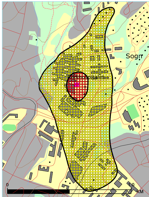
Figur 9-5. Støysoner i samsvar med retningslinje T-1442/2012. M 1:15 000.
