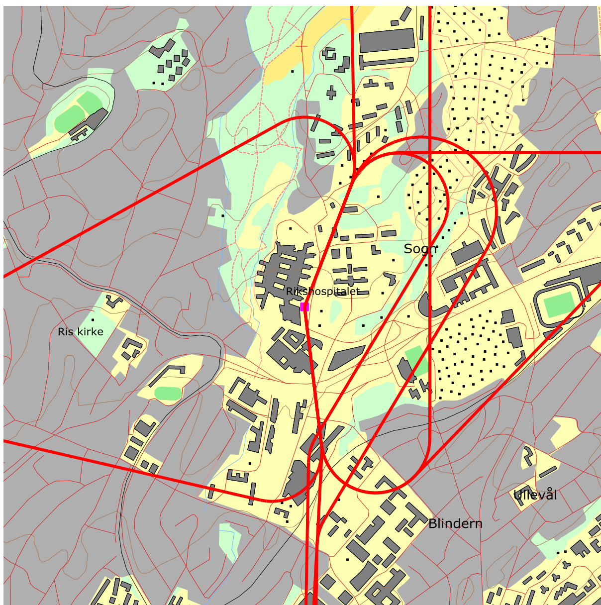
Figur 7-1. Traséer for landinger på Oslo helikopterlandingsplass Rikshospitalet. M 1:15 000.
