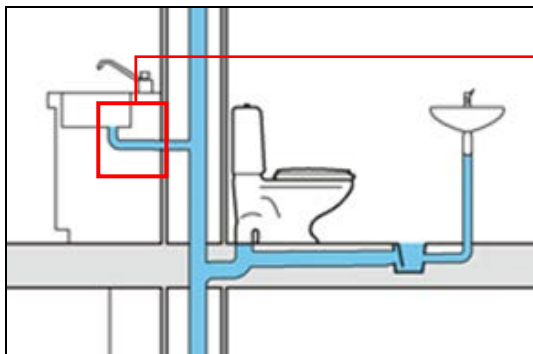
Fig. 55: 50 mm avløpsrør fra kjøkken
