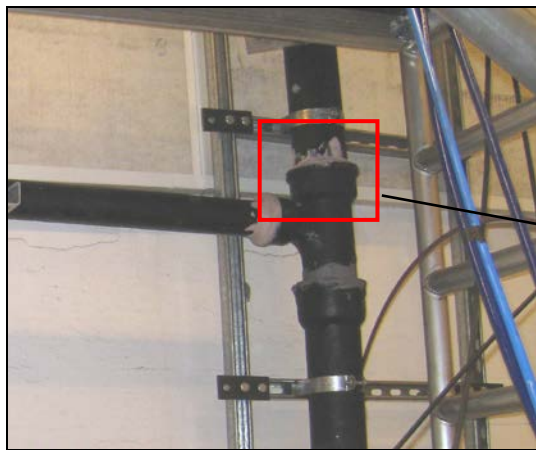
Fig. 77: Grenrør i støpejern
