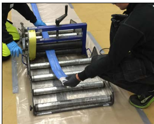
Fig. 11: Valsing av epoksy i strømpe for å fordele jevnt utover
