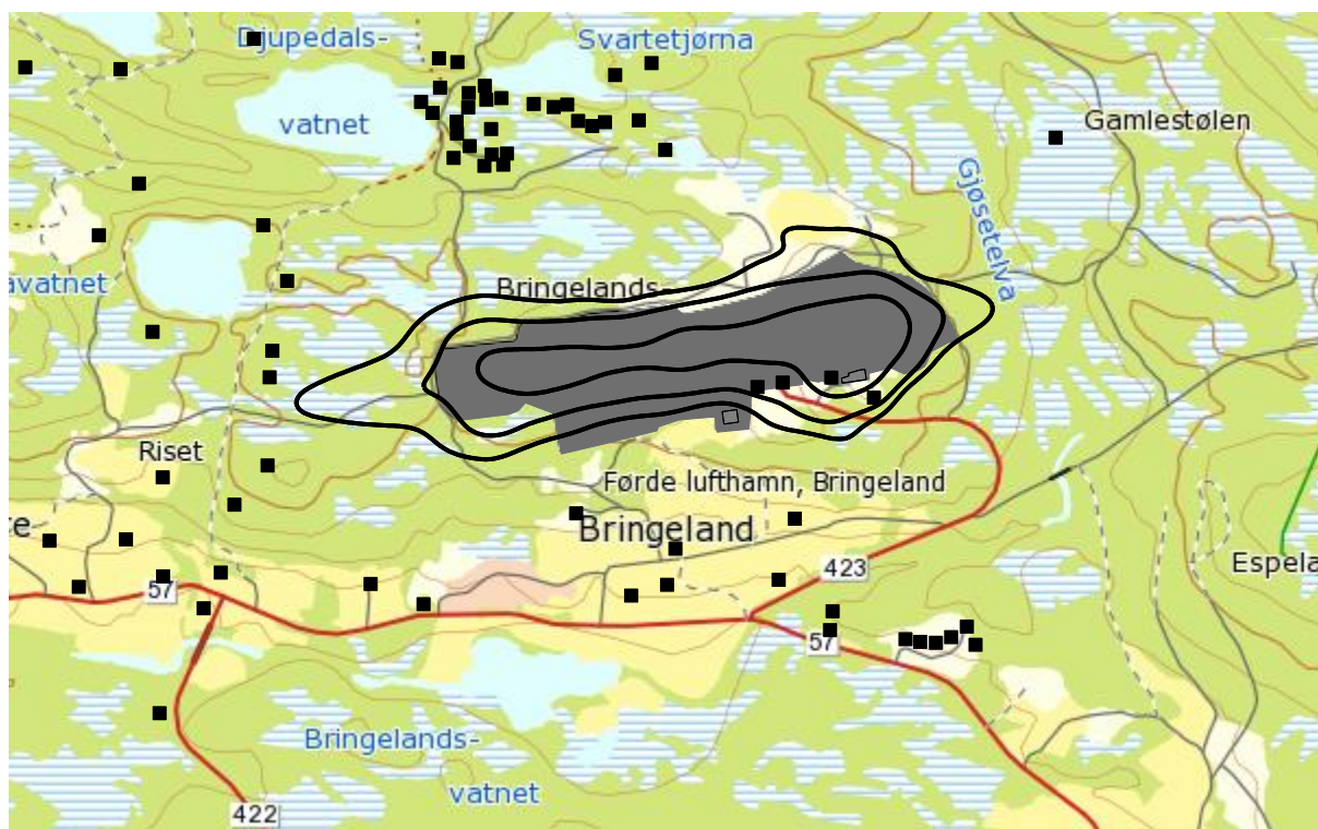
Figur 10-1. Kartleggingsgrenser for dagens situasjon. L_{Aeq24h} 51, 54 og 61 dBA. M 1:20 000.
