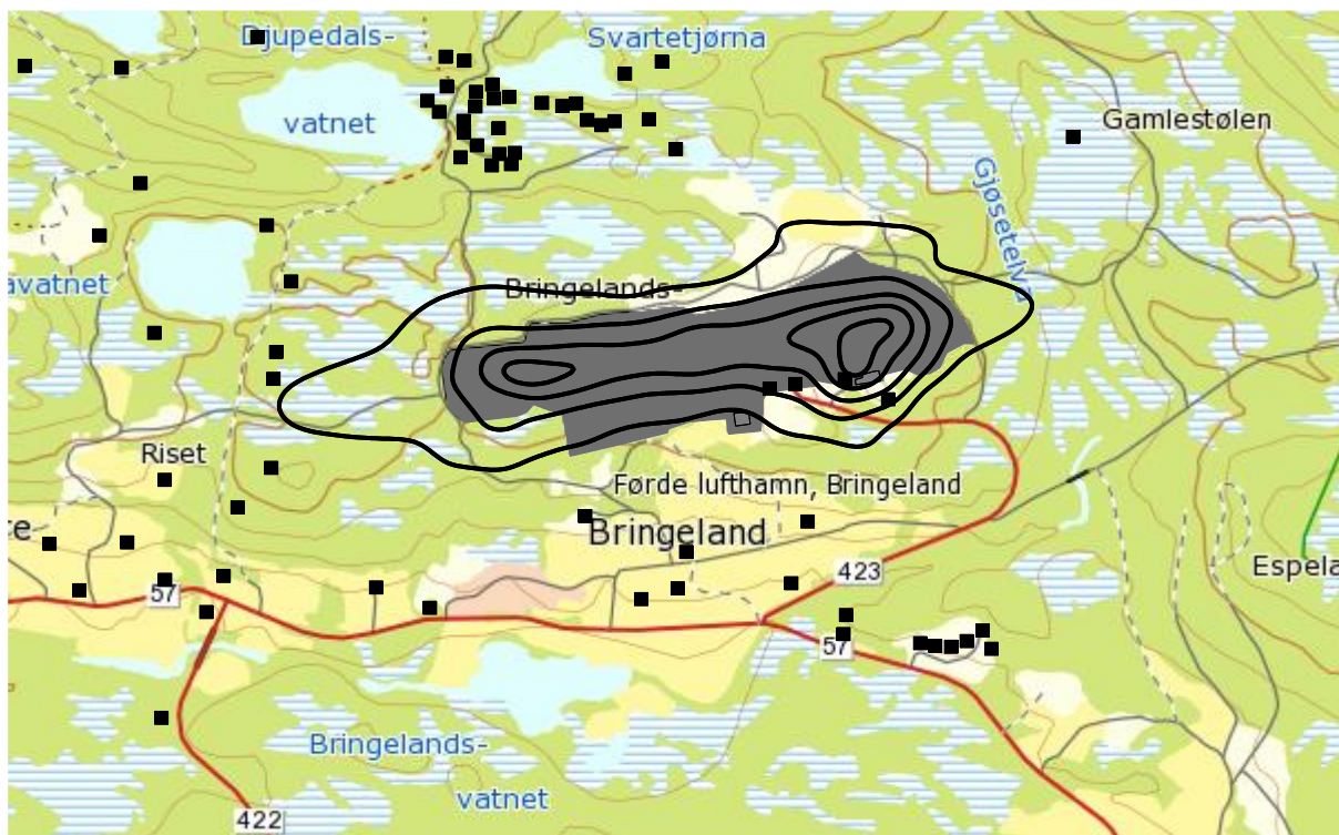
Figur 10-7. L_{Aeq24h} for dagens situasjon i 5 dB trinn fra 50 dBA. M 1:20 000.
