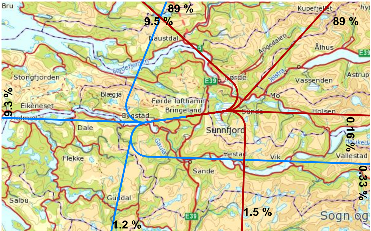
Figur 7-4. Traséer for landing (blå streker) og avgang (røde streker) på bane 07 med helikopter. M 1:400 000.
