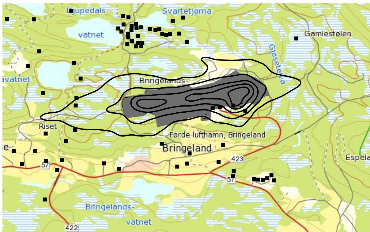
Figur 10-4. L_{den} for prognosesituasjonen i 5 dB trinn fra 50 dBA. M 1:20 000.
