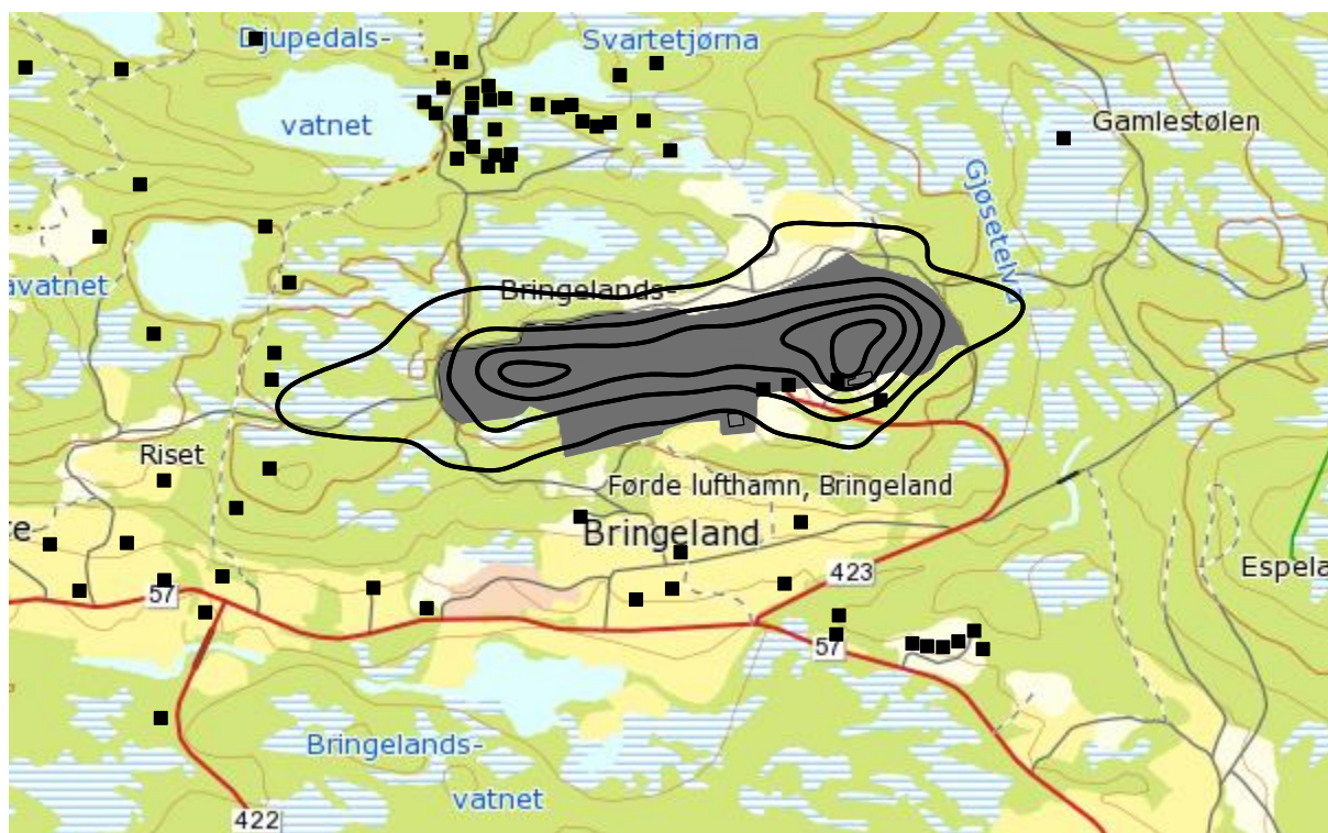
Figur 10-8. L_{Aeq24h} for prognosesituasjonen i 5 dB trinn fra 50 dBA. M 1:75 000.
