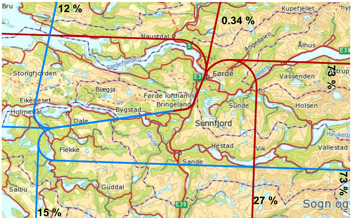
Figur 7-1. Traséer for landing (blå streker) og avgang (røde streker) på bane 07 med fly. M 1:400 000.
