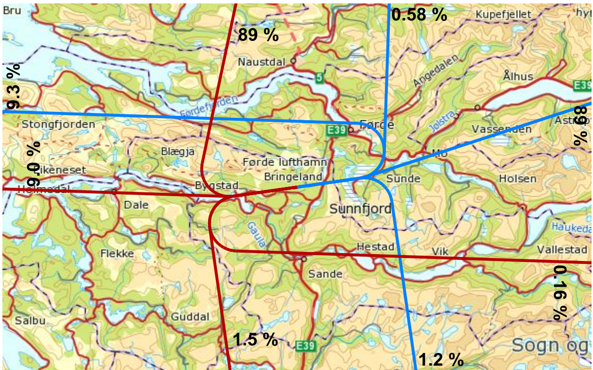
Figur 7-5. Traséer for landing (blå streker) og avgang (røde streker) på bane 25 med helikopter. M 1:400 000.
