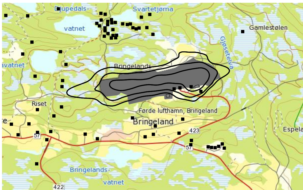
Figur 10-2. Kartleggingsgrenser for prognosesituasjonen. L_{Aeq24h} 51, 54 og 61 dBA. M 1:20 000.
