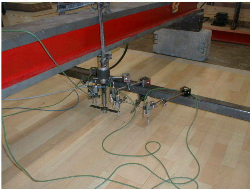
Fig. 14.2. Statistiske målinger for å bestemme nedbøyning og lastutbredelse for tynn parkett på elastisk underlag (36 mm trefiberplate). Punktlasten er påført midt på lamell og i lamellskjõt.
