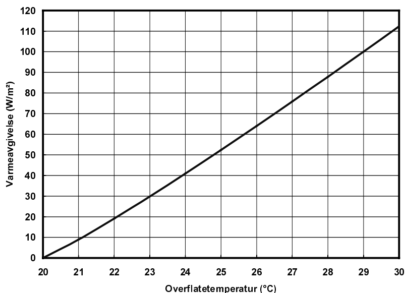
Fig. 3.1. Varmeavgivelse fra gulvvarmeanlegg som funksjon av gulvets overflatetemperatur. Romtemperaturen er 20 °C.
