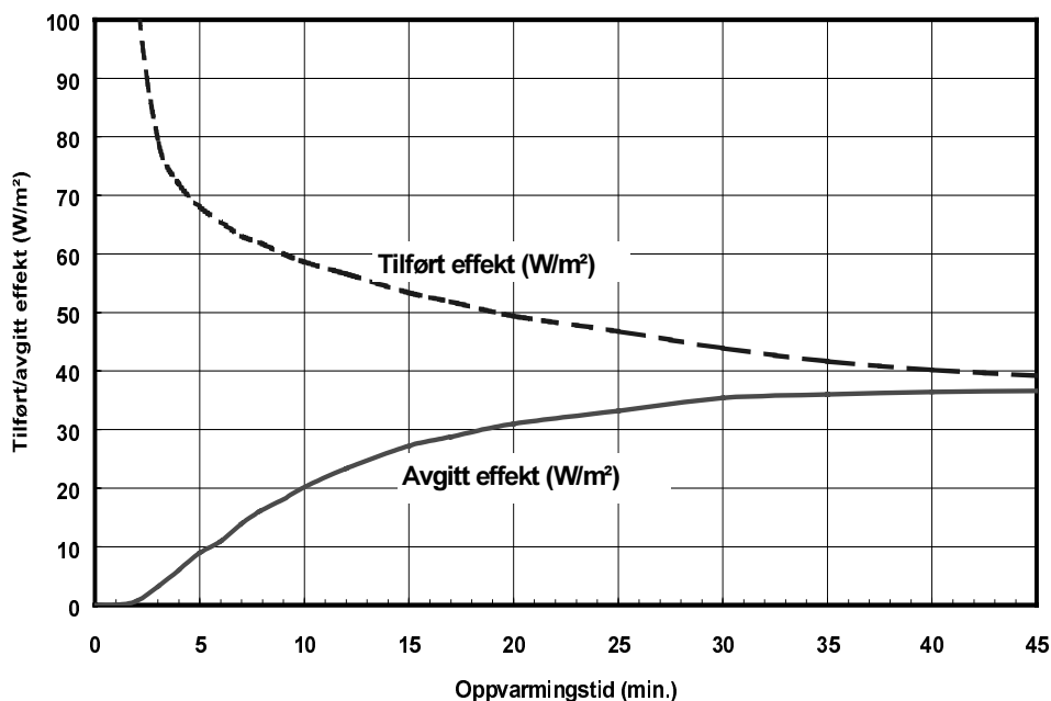
Fig. 15.8. Laboratiemålinger. Tilført og avgitt varme fra et vannbårent lett lavtemperatur gulvvarmeanlegg i en oppvarmingsperiode. Varmerørene ligger spor i fiberplater. Varmefordelingen besørges av Al-omega plater og gulvbelegget er 9 mm parkett. Middelttemperaturen er konstant ca. 30 °C og romtemperaturen 20 °C. Vannhastigheten er konstant 0,7 m/s.
