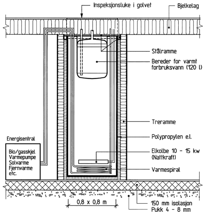
Fig. 9.1. Eksempel på trykløst varmelager, med volum ca. 1,5 m 3 i PP-plast. Varmelageret er integrert i bygningskonstruksjonen som inngår som del av tankens bæresystem.
