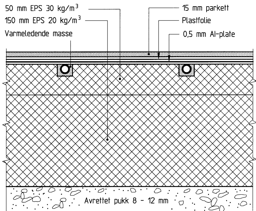
Fig. 12.2. Gulv på grunnen med gulvvarme. Varmereørene er lagt i spor i isolasjonen med godt ledende masse rundt varmereørene. Alternativt kan det brukes Al-plater med klips eller å forme Al-platen rundt røret ( \Omega -plater). På grunn av varmereørenes varmeisolerende egenskaper er god ledende kontakt mellom hele røroverflaten og aluminiumsplatene viktig for god varmeoverføring.
