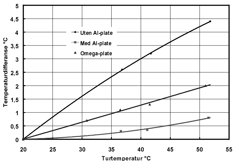
Fig. 12.5. Maksimal temperaturredifferanse på gulvoverflaten rett over og mellom varmerør. Det er brukt samme gulvoppbygging som i fig. 12.4.
