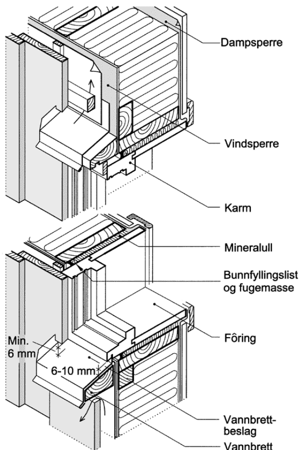
Figur 4.3 a Vindu satt inn i vegg med utlektet tømmermannskledning Vinduet kan eventuelt settes lenger ut i vegg slik at overligger danner sidelist (Byggdetaljer 523.701).
