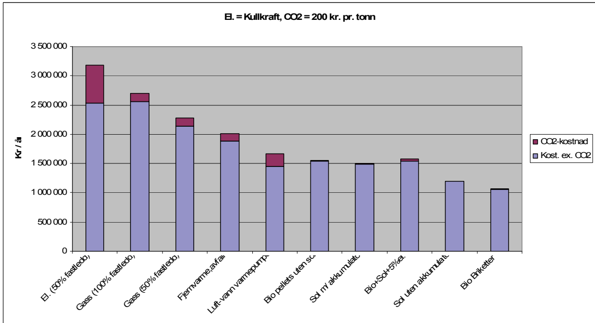
FIGUR 7-6 Årlige energikostnader der for de ulike varmealternativene med kalkylerente på 3 %. En CO 2 -kostnad på 200 kr/tonn er vist på toppen (mørke rødt) av vanlige energikostnader (blå). CO 2 utslipp fra el er regnet med kommer fra kullkraftverk.
