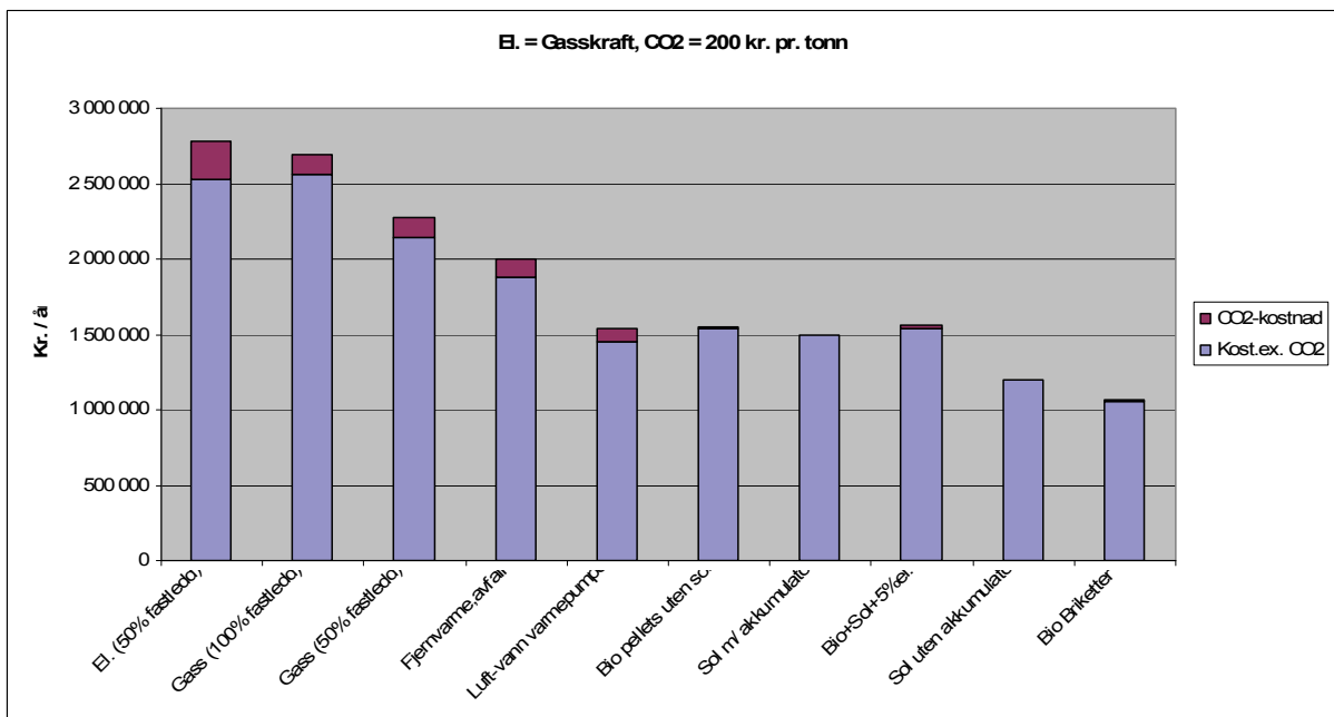
FIGUR 7-7 Årlige energikostnader der for de ulike varmealternativene med kalkylerente på 3 %. En CO 2 -kostnad på 200 kr/tonn er vist på toppen (mørke rødt) av vanlige energikostnader (blå). CO 2 utslipp fra el er regnet med kommer fra gasskraftverk.
