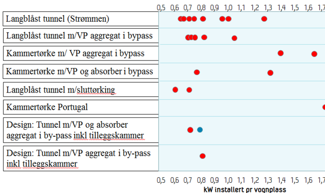
Figur 5: Oversikt over installert effekt pr vognplass for ulike teknologiløsninger i klippfisknæringen
