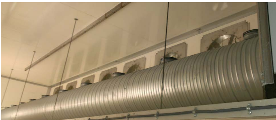
Figur 6: Ventilasjonsrør med flere åpninger kan være en mulighet til å distribuere oppvarmet uteluft i et større egnet lager for slutt-tørking (ikke med viftene bak).
