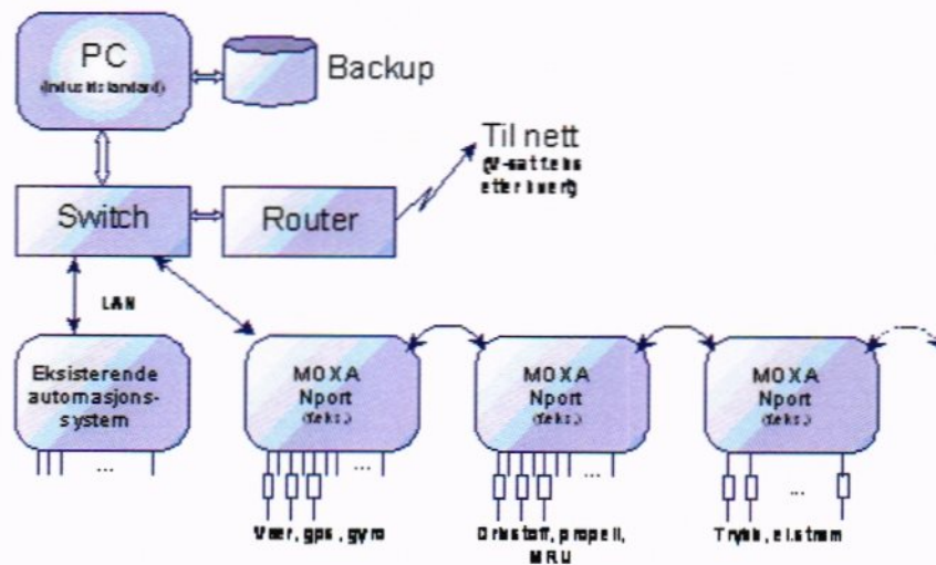
Figur 2. Prinsippskisse av instrumentering med nettverk.
