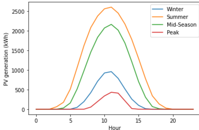
Figur 7. Timeprofiler av solceller produksjon for et døgn i forskjellige sesonger i 2050 for hele Furuset.
