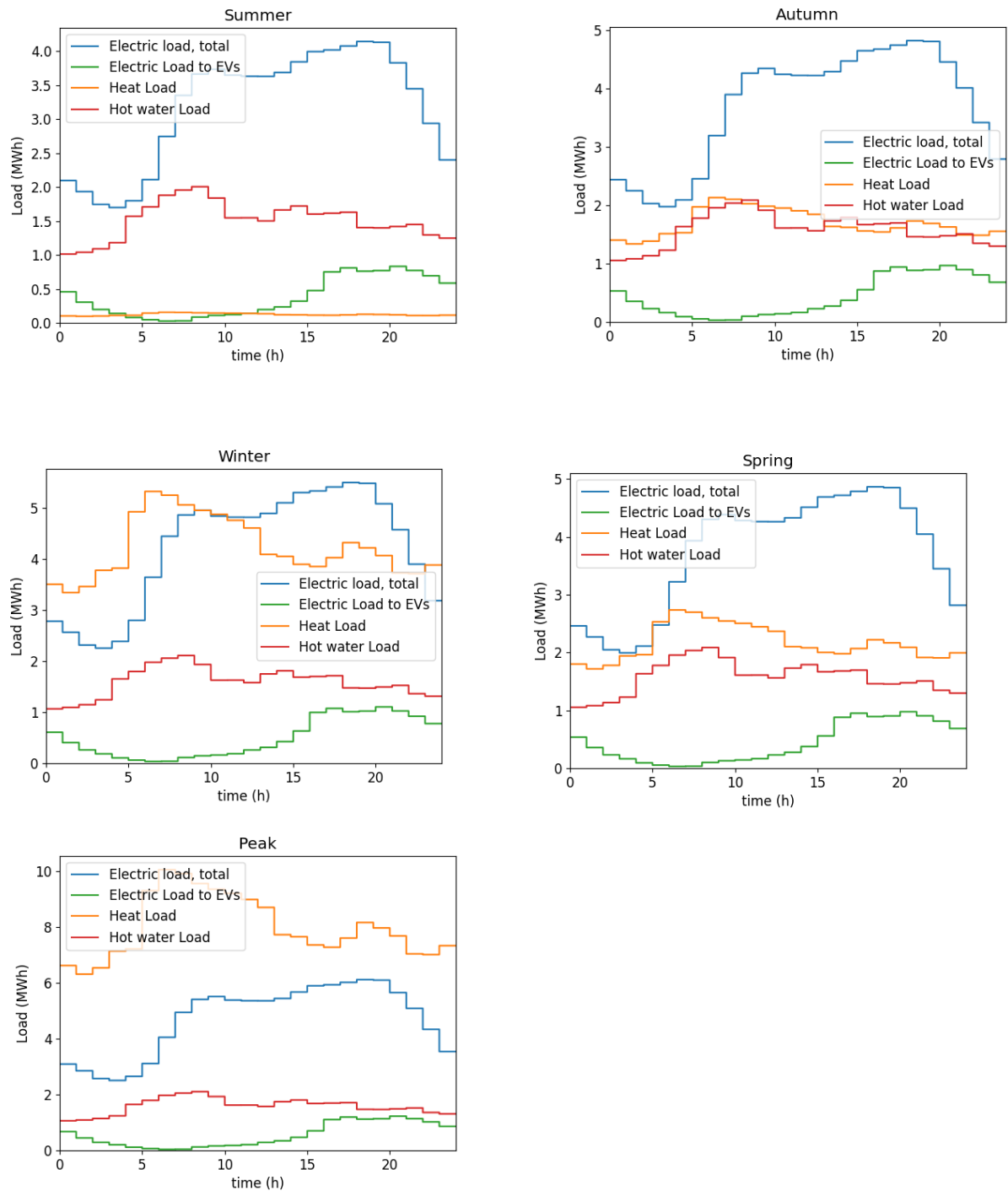
Figur 6. Døgnprofiler for det totale energibehovet på Furuset for de ulike sesongene, fordelt til totalt strømspesifikt behov, strømbehov til ladning av elbiler, romoppvarmingsbehov og varmtvannsbehov.
