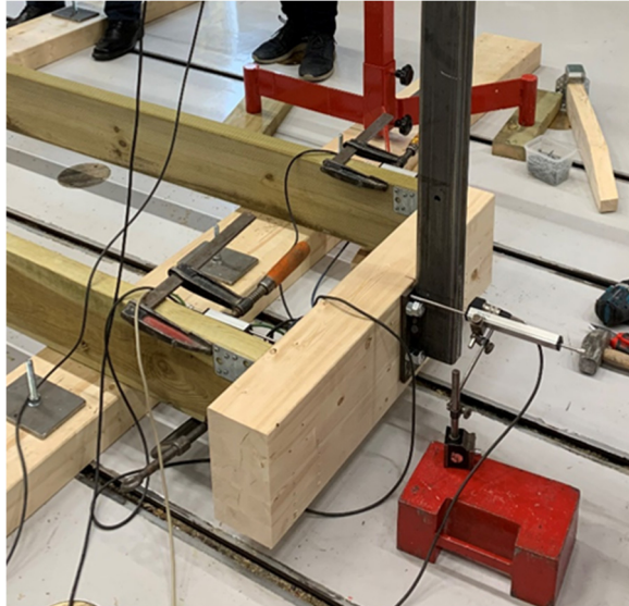
Figur 38 Prøveoppstilling H, test 16
