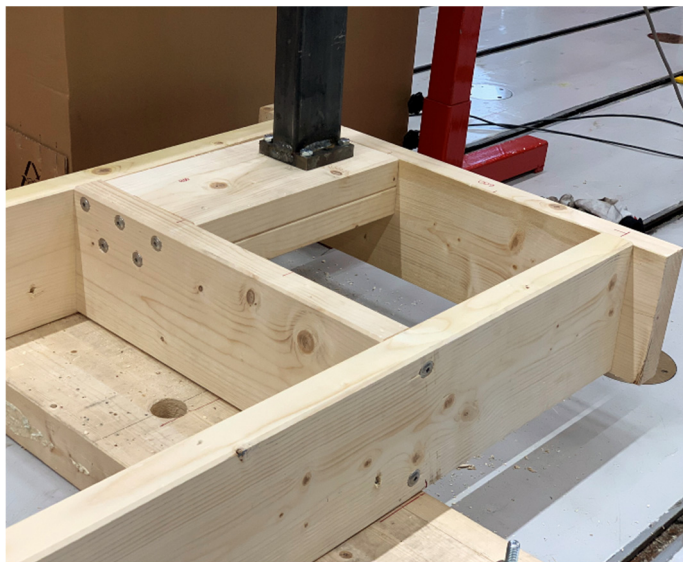
Figur 65 Prøveoppstilling S, test 42. Konstruksjonen består av 48 mm x 198 mm konstruksjonsvirke og er i hovedsak skrudd sammen av 8x120 mm treskruer med stort hode.
