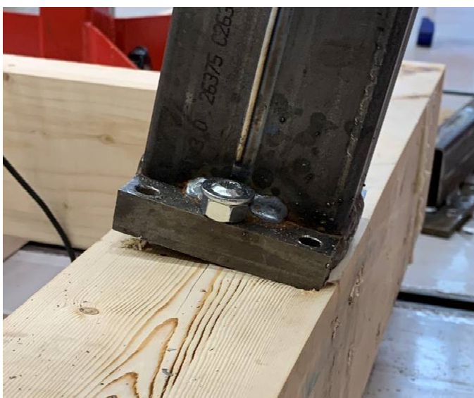
Figur 54 Prøveoppstilling O. Toppmontert stolpe festet med bare to skruer i midten. Stor deformasjon ved 1,0 kN.
