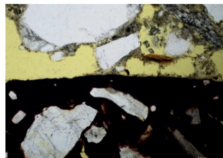
FIGUR 1. Tynnslianalyse av heftsoner mellom teglstein (nede mørke del) og murmørtel. Gule felt markerer luftporer. Analyse og foto: Marit Haugen, SINTEF Byggforsk.
