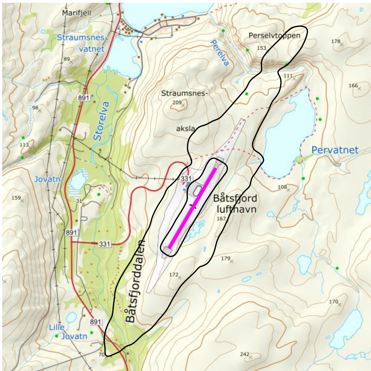
Figur 9-4. L_{den} 40 og 50 dBA for prognosesituasjonen (2028). M 1:25 000.
