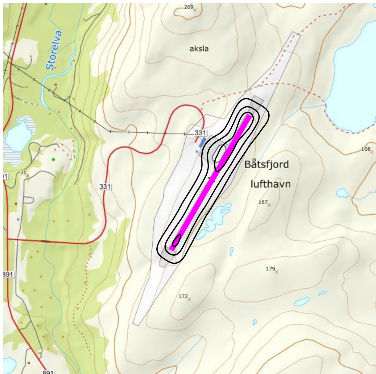
Figur 10-3. L_{den} for dagens situasjon (2017) i 5 dB trinn fra 50 dBA. M 1:15 000.
