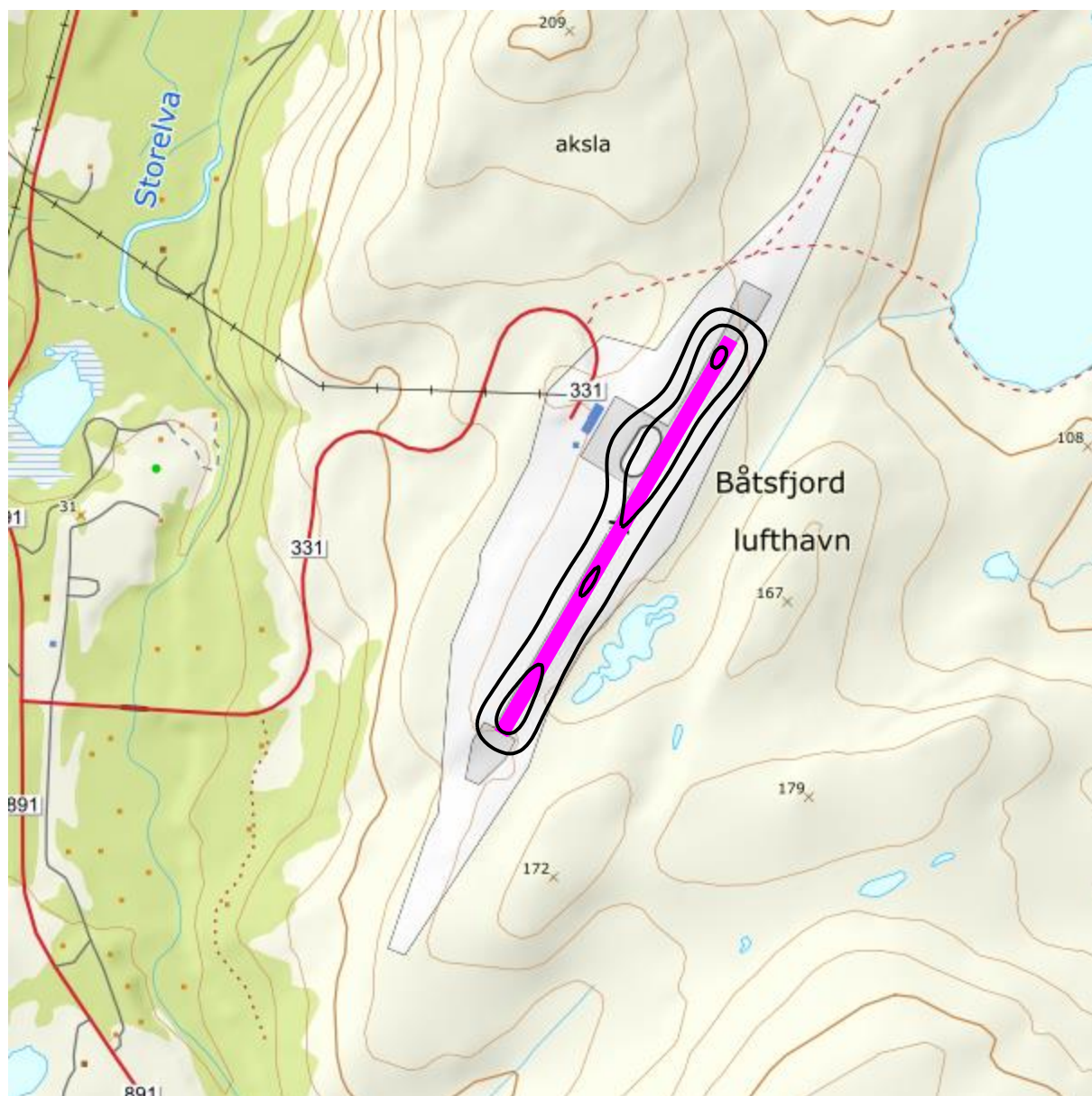
Figur 10-7. L_{Aeq24h} for dagens situasjon (2017) i 5 dB trinn fra 50 dBA. M 1:15 000.
