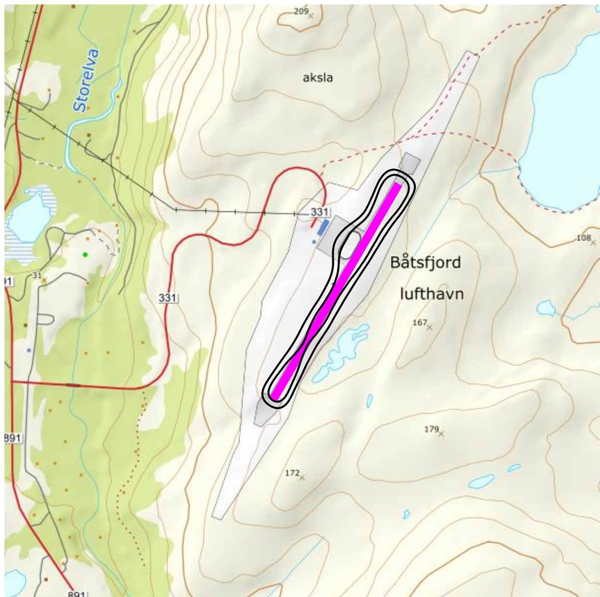
Figur 10-1. Kartleggingsgrenser for dagens situasjon (2017). L_{Aeq24h} 51 og 54 dBA. M 1:15 000.
