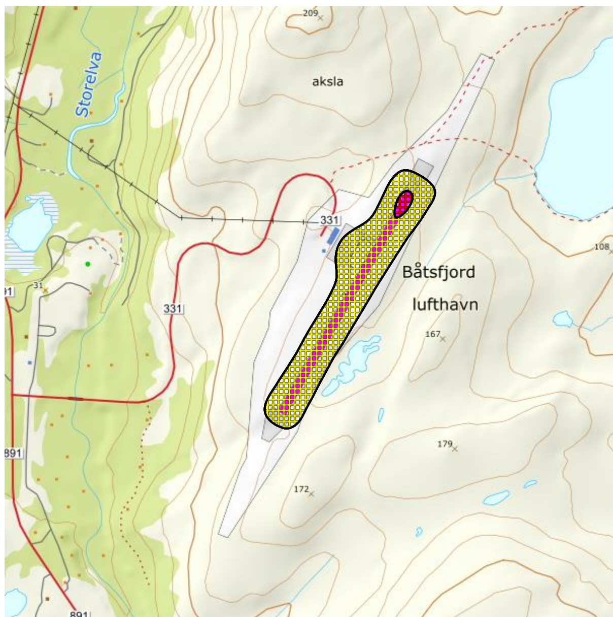
Figur 9-1. Rød og gul støysone for Båtsfjord lufthavn for dagens situasjon (2017). M 1:15 000.
