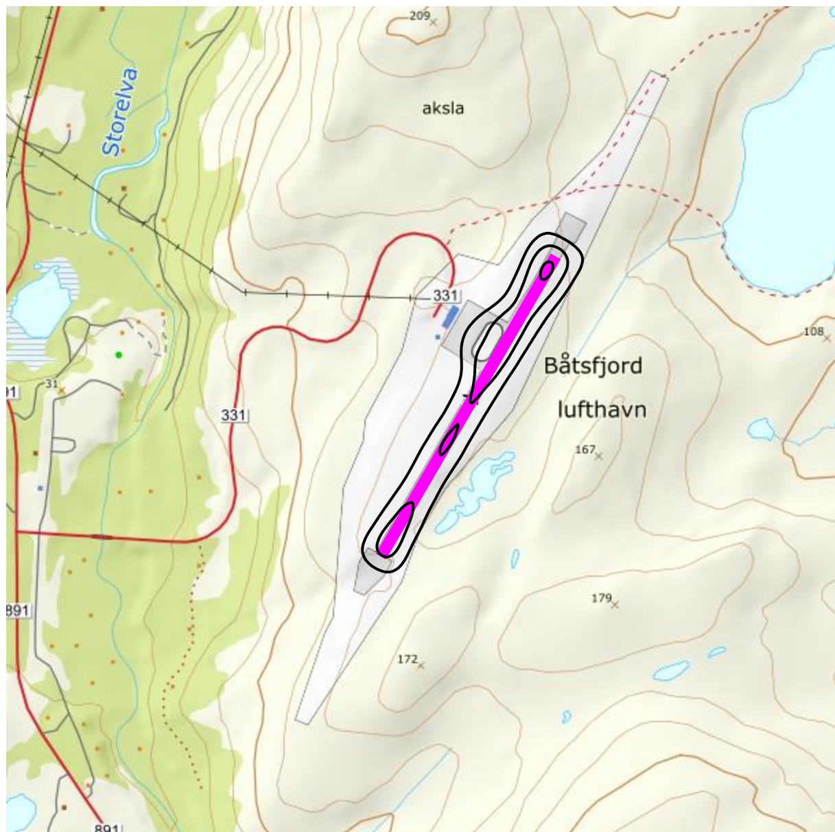
Figur 10-8. L_{Aeq24h} for prognosesituasjonen (2028) i 5 dB trinn fra 50 dBA. M 1:15 000.
