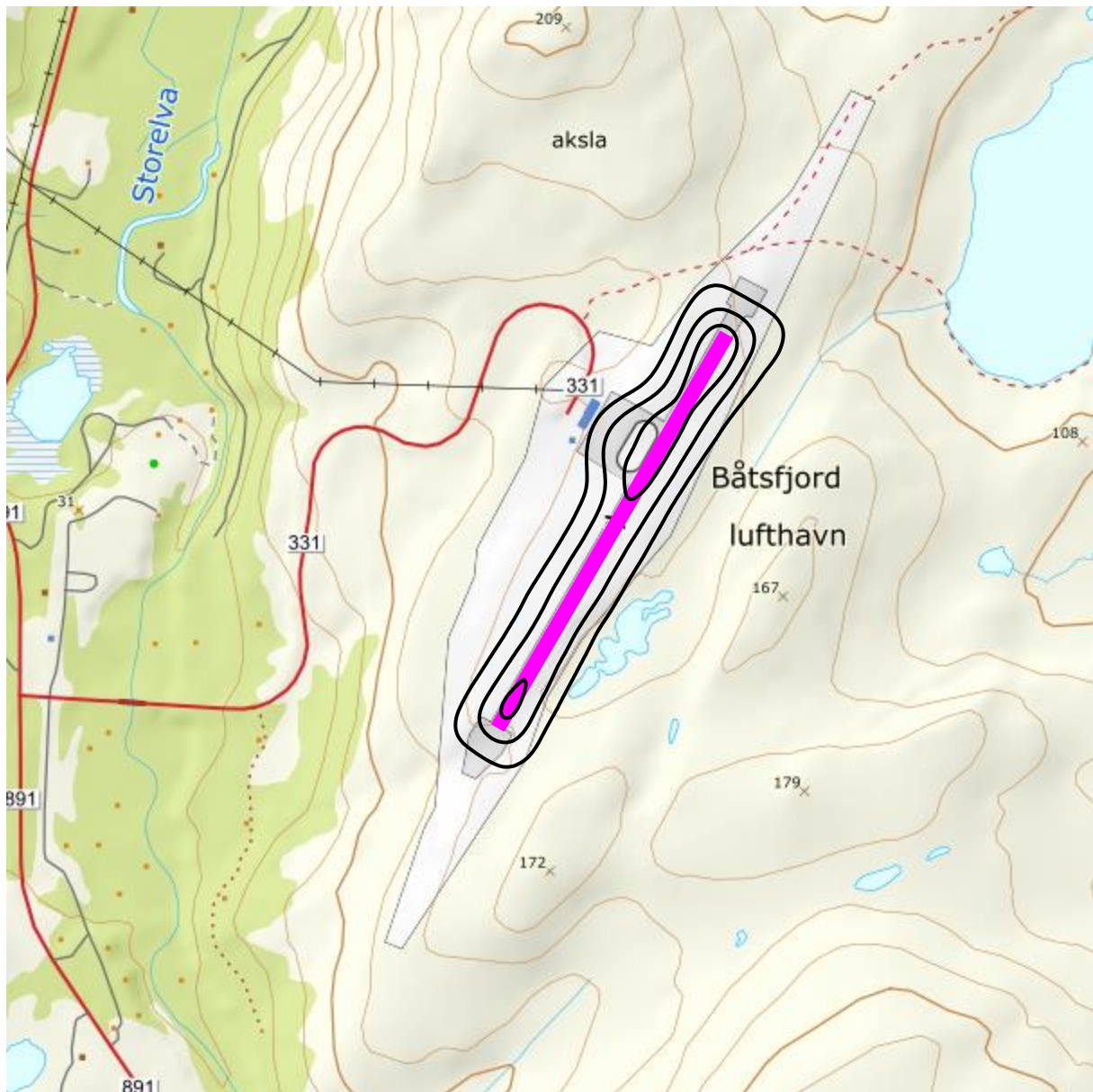
Figur 10-4. L_{den} for prognosesituasjonen (2028) i 5 dB trinn fra 50 dBA. M 1:15 000.
