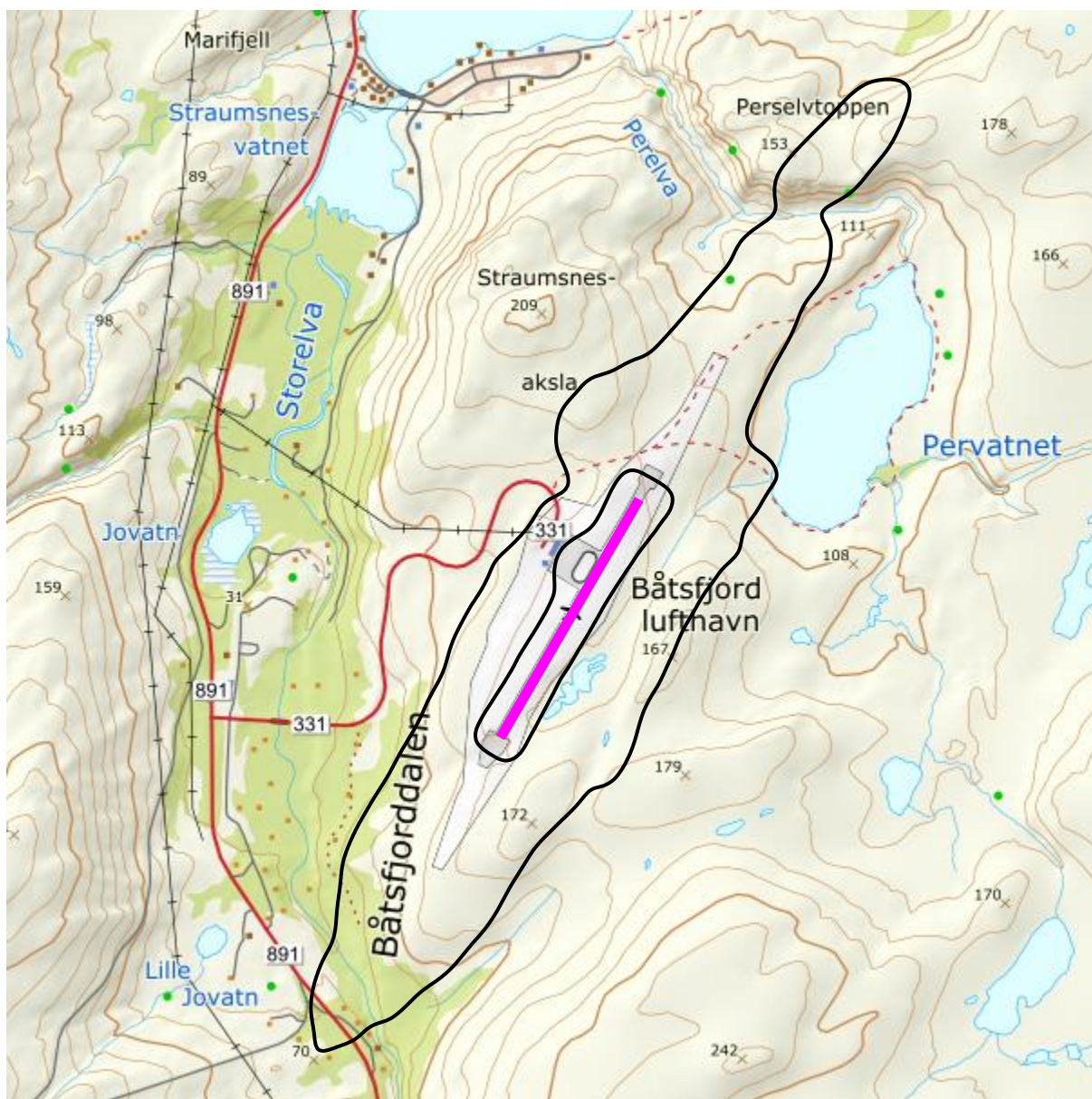
Figur 9-3. L_{den} 40 og 50 dBA for dagens situasjon (2017). M 1:25 000.
