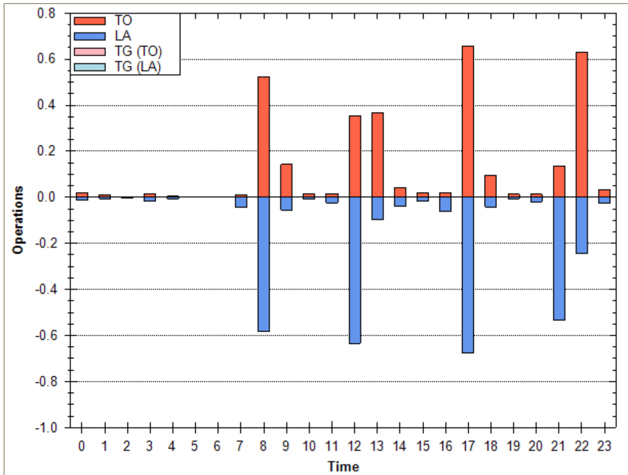
Figur 6-1. Antall flybevegelser per time for et gjennomsnittsdøgn i 2017.
