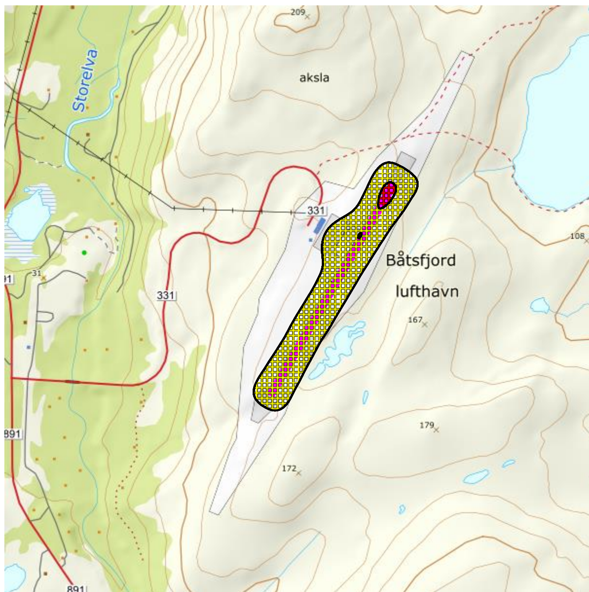
Figur 9-2. Rød og gul støysone for Båtsfjord lufthavn for prognosesituasjonen (2028). M 1:15 000.
