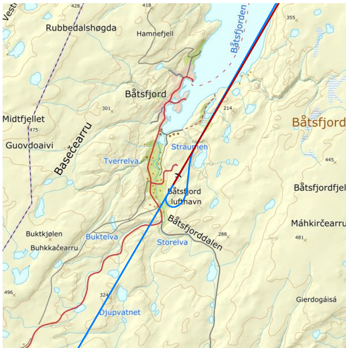
Figur 7-1. Traséer for landing (blå strek) og avgang (rød strek) på bane 03. M 1:100 000.
