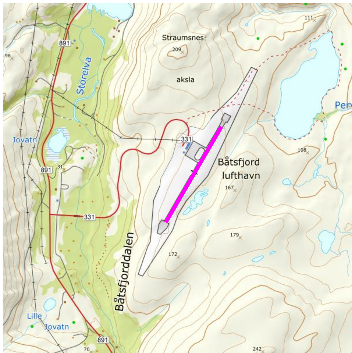
Figur 5-1. Båtsfjord lufthavn med omgivelser. Rullebanen (terkel til terskel) er markert rosa. M 1:20 000.
