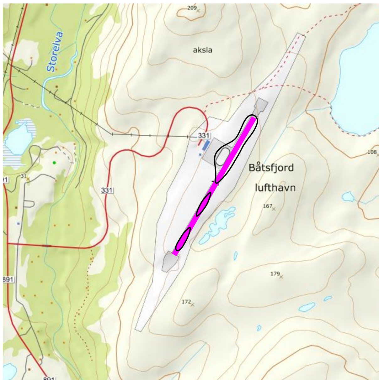
Figur 10-5. L_{\text{night}} for dagens situasjon (2017) i 5 dB trinn fra 50 dBA. Det er så lite trafikk på natt at bare koten for 50 dBA er definert. M 1:15 000.
