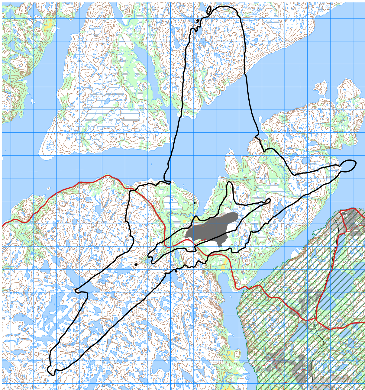
Figur 9-5. L_{den} 40 og 50 dBA for prognosesituasjonen (2027). M 1:100 000.
