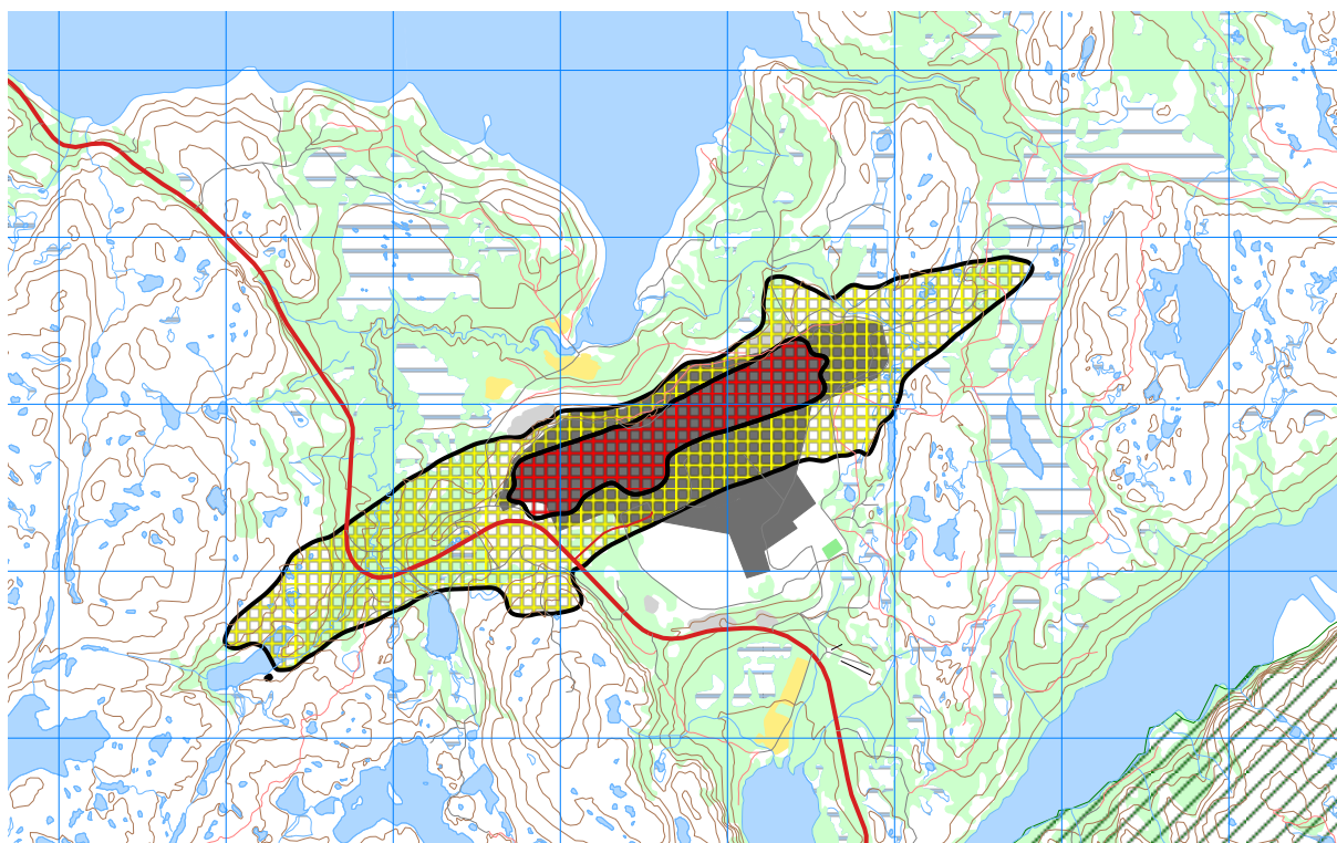
Figur 9-1. Rød og gul støyzone for Kirkenes lufthavn for dagens situasjon (2016). M 1:50 000.
