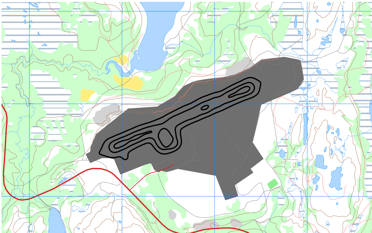
Figur 10-6. L_{\text{night}} for prognosesituasjonen (2027) i 5 dB trinn fra 50 dBA. Det er så lite trafikk på natt at bare kotene for 50, 55, og 60 dBA er definert. M 1:25 000.
