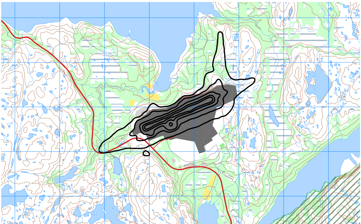
Figur 10-8. L_{Aeq24h} for prognosesituasjonen (2027) i 5 dB trinn fra 50 dBA. M 1:50 000.
