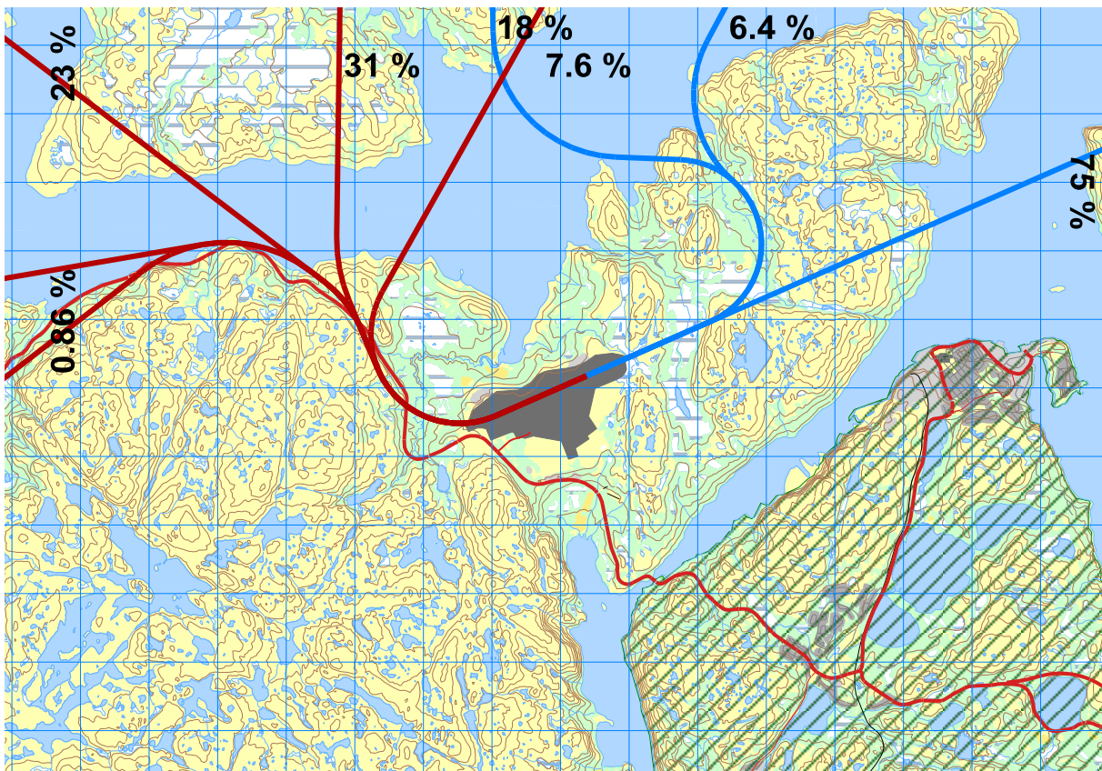
Figur 7-5. Traséer for avganger (rød) og landinger (blå) på bane 24 med turboprop. M 1:100 000.
