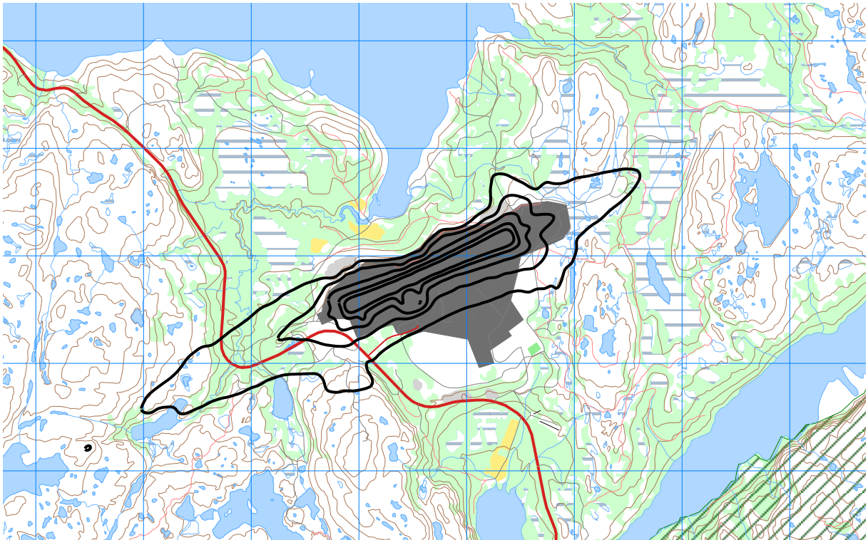
Figur 10-7. L_{Aeq24h} for dagens situasjon (2016) i 5 dB trinn fra 50 dBA. M 1:50 000.
