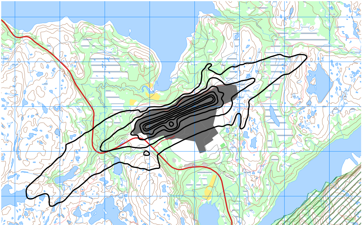
Figur 10-3. L_{den} for dagens situasjon (2016) i 5 dB trinn fra 50 dBA. M 1:50 000.
