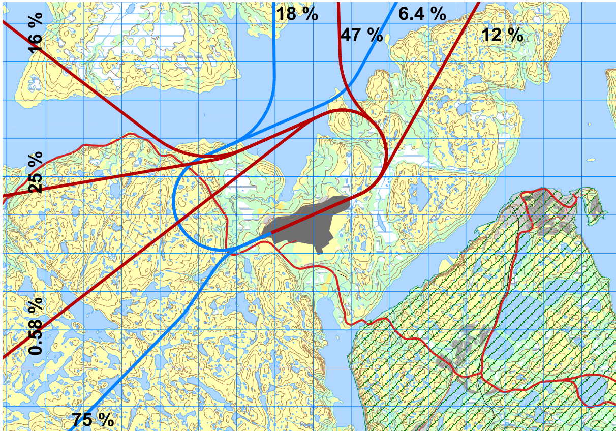
Figur 7-4. Traséer for avganger (rød) og landinger (blå) på bane 06 med turboprop. M 1:100 000.
