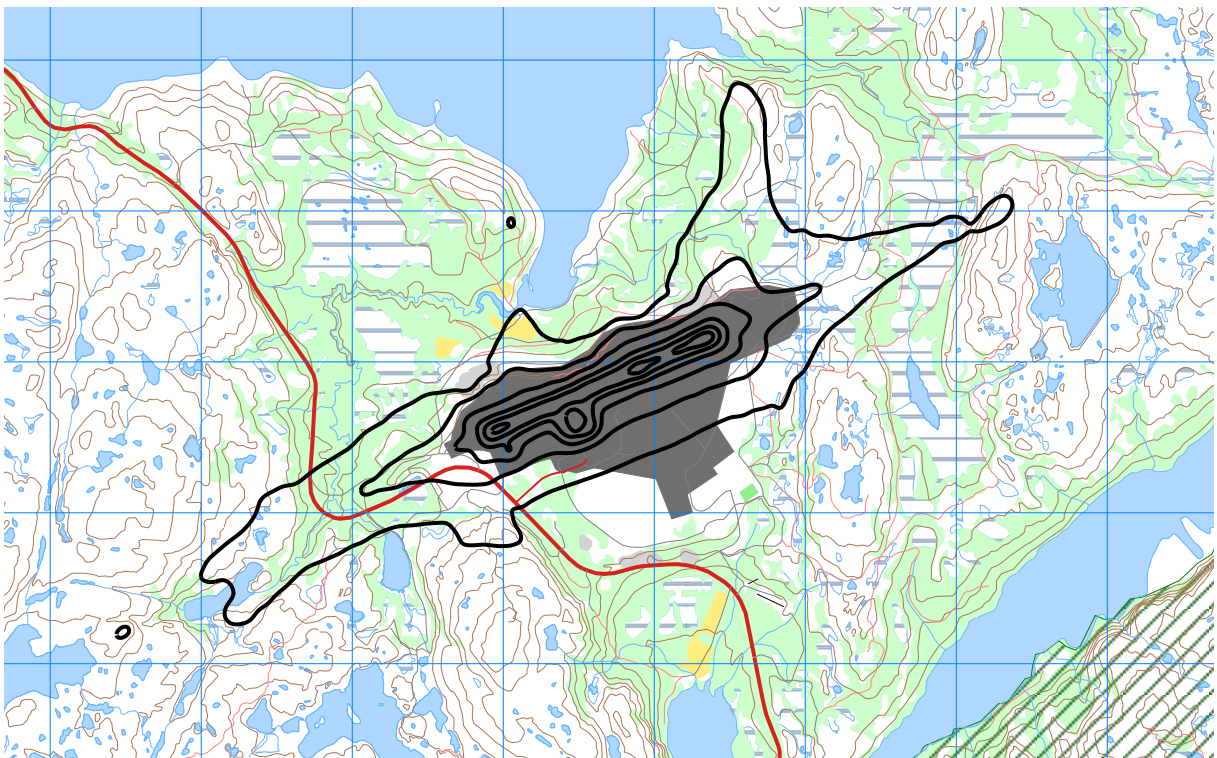
Figur 10-4. L_{den} for prognosesituasjonen (2027) i 5 dB trinn fra 50 dBA. M 1:50 000.
