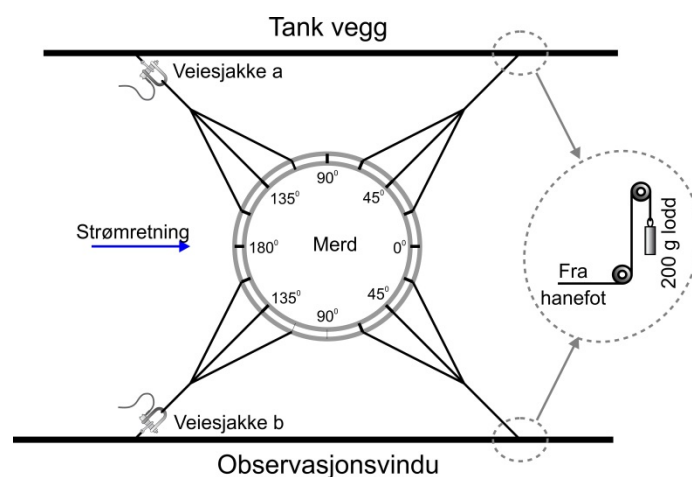
Figur 5. Oppsett av merd med veiesjakkler oppstrøms og forspenning av merden nedstrøms.
