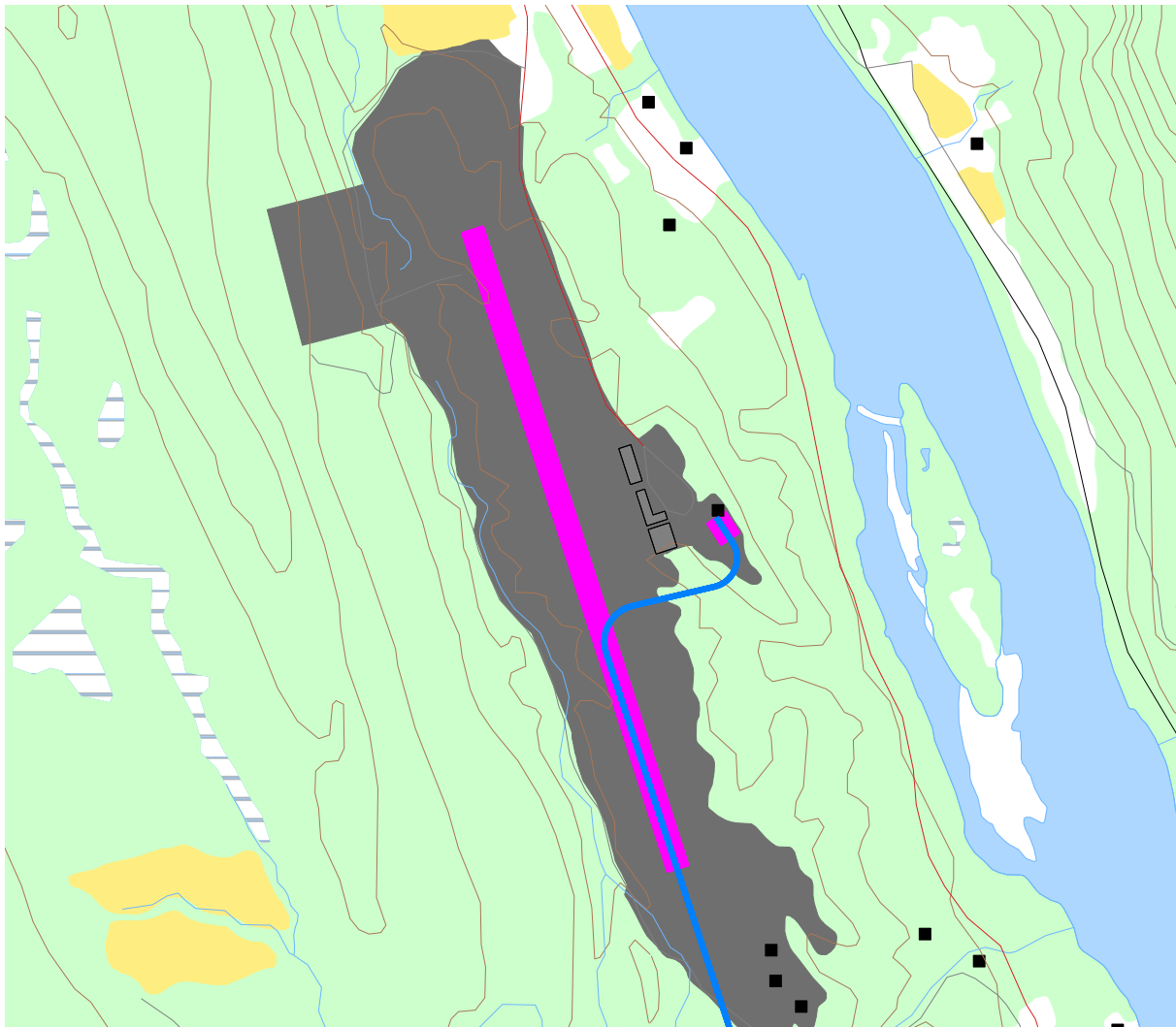
Figur 7-9. Skisse over siste delen av landing over bane 34 med helikopter. M 1:10 000.
