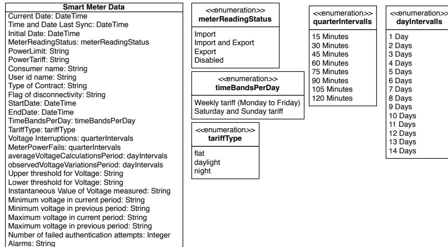
Fig. 4. Smart Meter Data Structure
