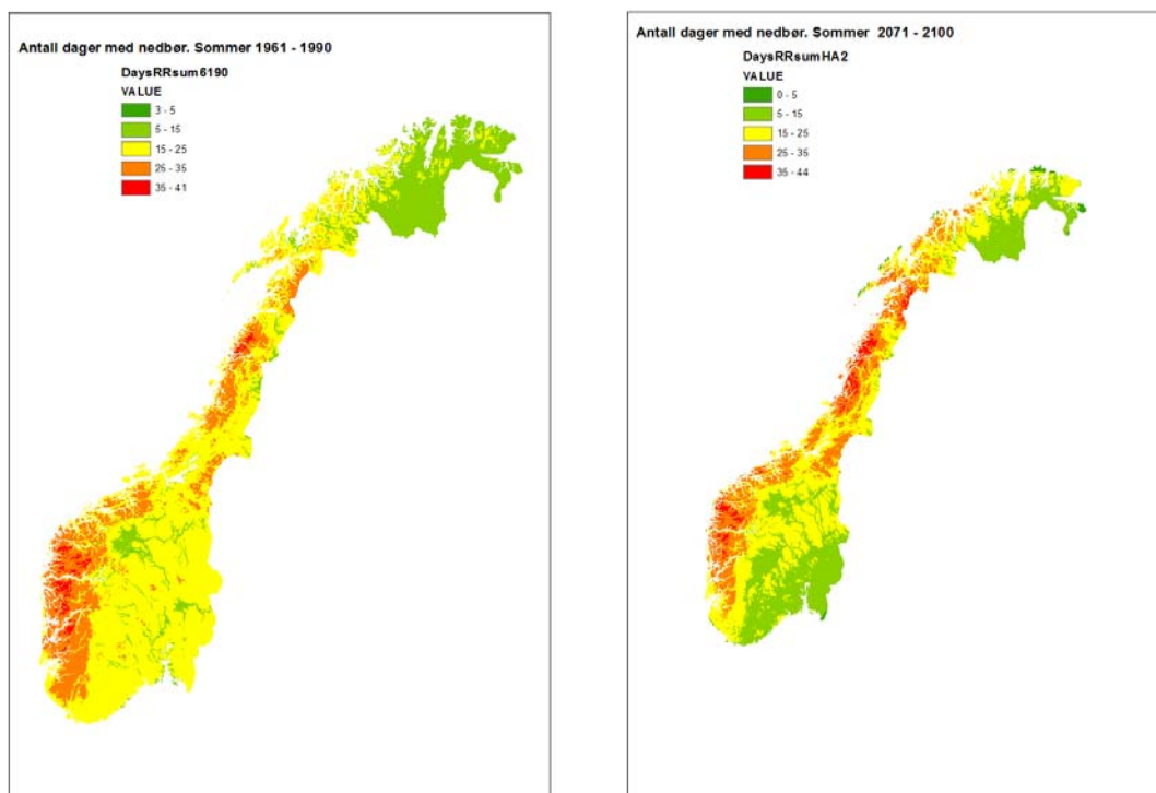
Figur 6.2.4 b Antall dager med sommernedbør (> 5 mm) for normalperioden 1961-1990 og for scenario 2071-2100
