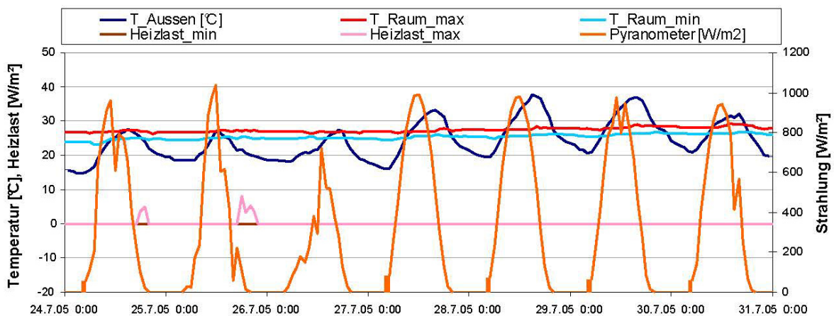
Figur 10: Ute- og innetemperatur på en varm og solrik sommerdag (rødt: innetemperatur leilighet maks, lyseblått: innetemperatur leilighet min., brun: oppvarming min., rosa: oppvarming maks, mørkeblått: utetemperatur, oransje: solinnstråling)
