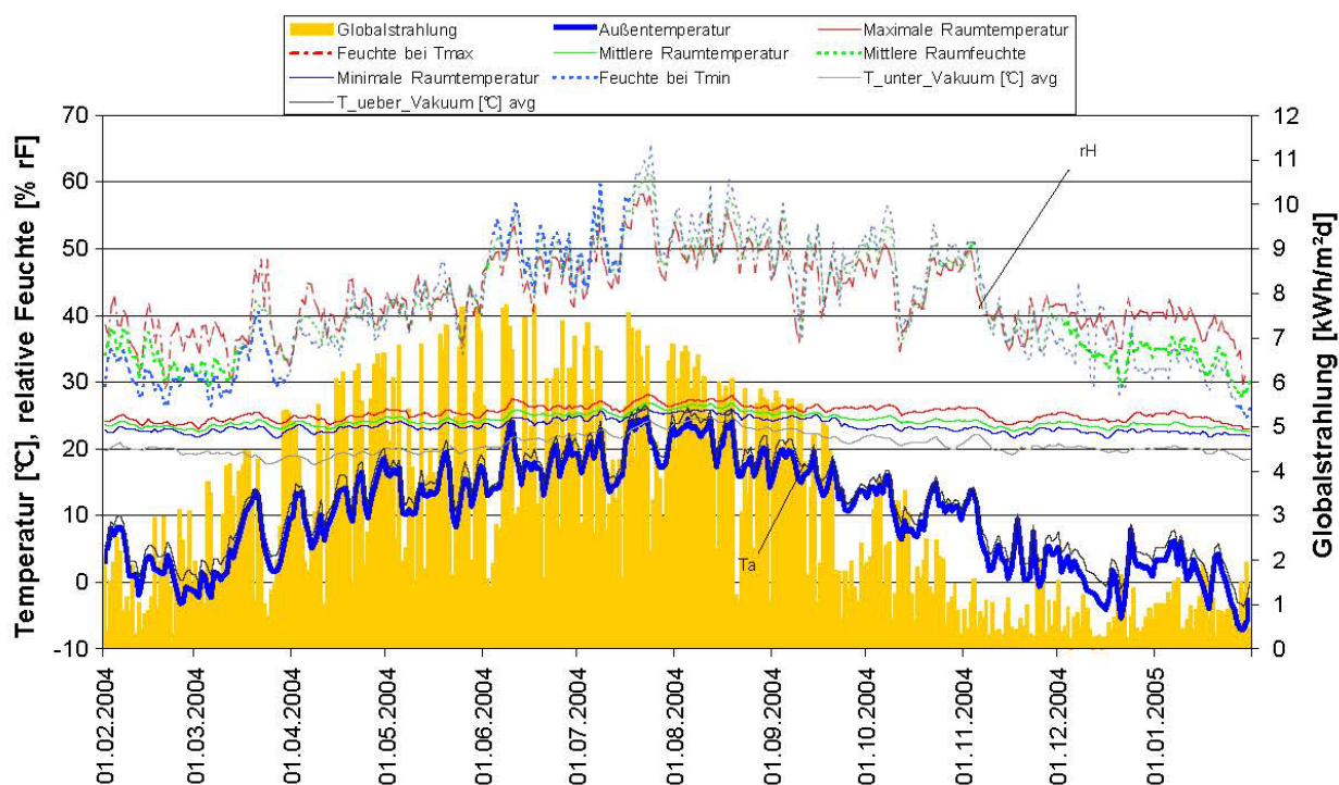
Figur 8: Inneklima Solarcity Linz første mål-året feb 2004 – jan 2005. (blått, tykk linje: utetemperatur, rødt, grønn, blått, grått: innetemperatur i leilighetene, gult: solinnstråling, stiplede linjene: luftfuktighet)
