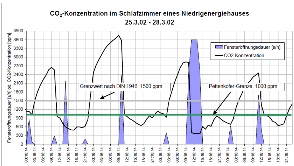
Figur 14: CO 2 -konsentrasjon på soverommet i en lavenergibolig med fuktstyrt avtrekksventilasjon (svart kurve viser CO 2 -konsentrasjon, lilla felter viser perioder for vindusluffing)
