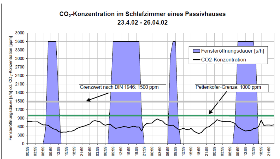
Figur 15: CO 2 -konsentrasjon på soverommet i en passivhusbolig med balansert ventilasjon (svart kurve viser CO 2 -konsentrasjon, lilla felter viser perioder for vindusluffing)
