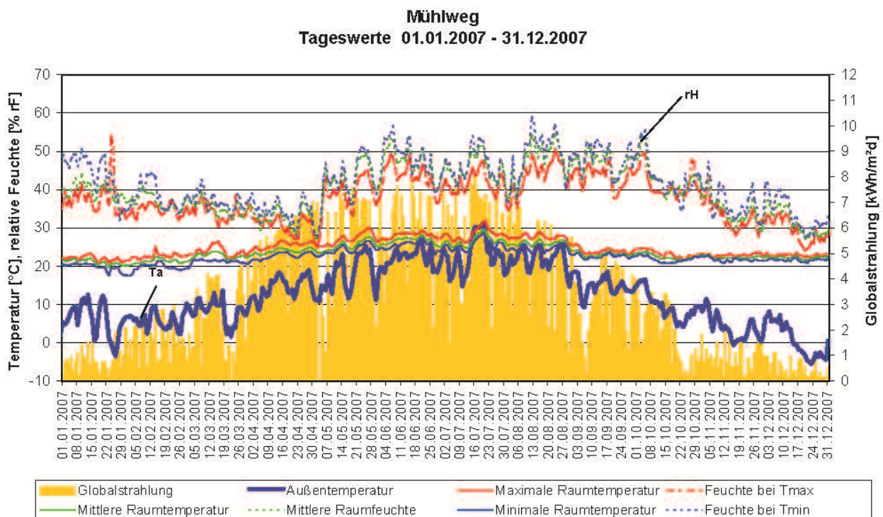
Figur 4: Romtemperatur og utetemperatur første målåret (blått, tykk linje: utetemperatur, rødt, grønn, blått, grått: innetemperatur i leilighetene, gult: stråling, stiplede linjer: luftfuktighet)
