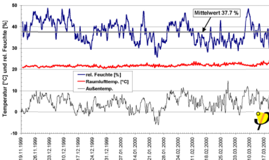
Figur 19: Målinger av relative romluftfuktighet (blå kurve), romtemperatur (rød kurve), sett i forhold til utetemperaturen (svart kurve).
