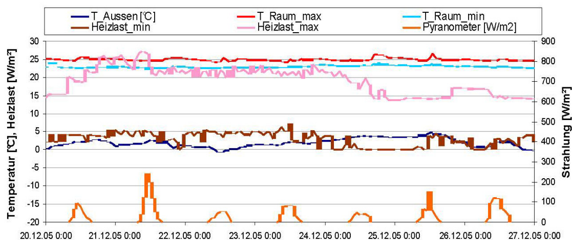
Figur 11: Ute- og innetemperatur på en overskyet uke om vinteren (rødt: innetemperatur leilighet maks, lyseblått: innetemperatur leilighet min., brun: oppvarming min., rosa: oppvarming maks, mørkeblått: utetemperatur, oransje: solinnstråling)
