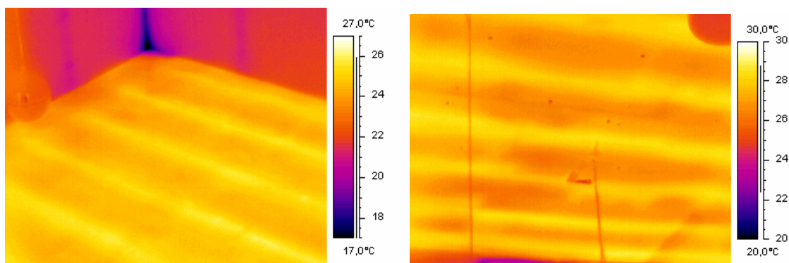
Figur 4.11: Temperaturfordelingen over gulvflaten (t.v.) og takflaten (t.h.).
