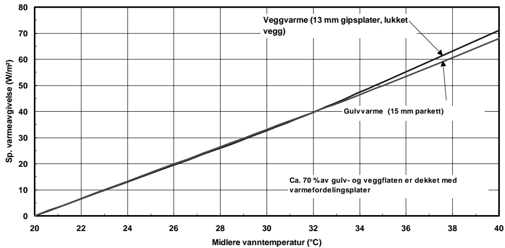
Fig. 7.1.3. Spesifikk varmeavgivelse fra et vannbåren gulv- og veggvarme i en innervegg. Veggghøyden er 2,4 m og veggen er dekket med gipsplater på begge sider. Gulvbelegget er 15 mm parkett.
