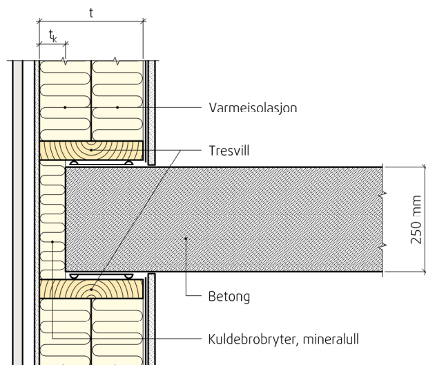
Figur 37. Kuldebroverdi for yttervegg av bindingsverk av tre mot etasjeskiller av betong. Konduktiviteten til betong er variert fra 1,65 til 2,3 W/mK.
