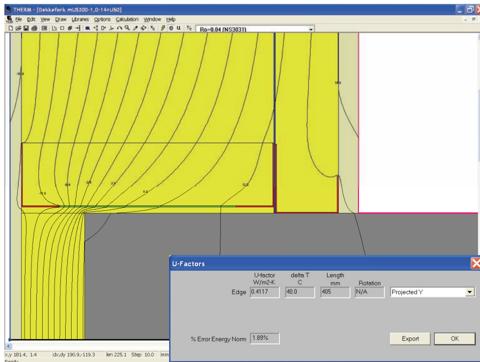
Figur 5. Figur av beregningsmodellen i THERM, med beregnet U-verdi. Her er det antatt at skumlist under bunnsvill er sammenpresset til 5 mm med \lambda = 0,037 \text{ W/mK} .
