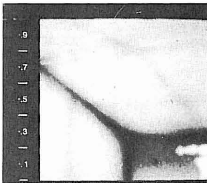
Loftsbjelkelag isolert med innblåsning av steinull. Termogram viser feilfri isolasjon i taket.
