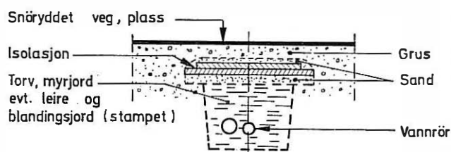
SNITT B-B
