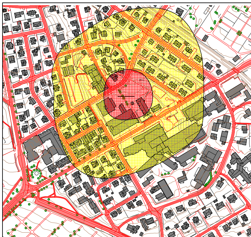
Figur 5-1 Støysoner for midlertidig landingsplass ved Tønsberg Sykehus. M 1:5 000.
