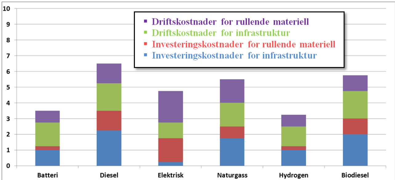
Figur 24: Estimerer for forventet Totalkostnad for de ulike konseptene, fordelt på investerings- og driftskostnader. Kostnader for batteri- og hydrogenkonseptene forventes å falle betydelig i årene som kommer.
