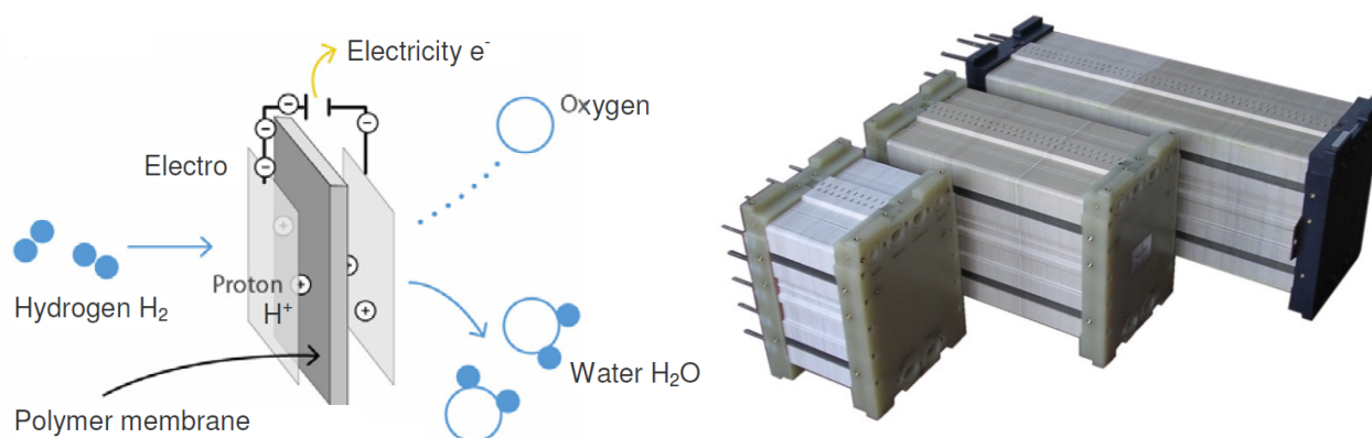
Figur 11: Prinsippet for en brenselcelle (til venstre) og eksempler på cellestaker (til høyre) der opp til noen hundre celler er satt sammen for at enheten skal gi den spenning og strøm som applikasjonen krever.
