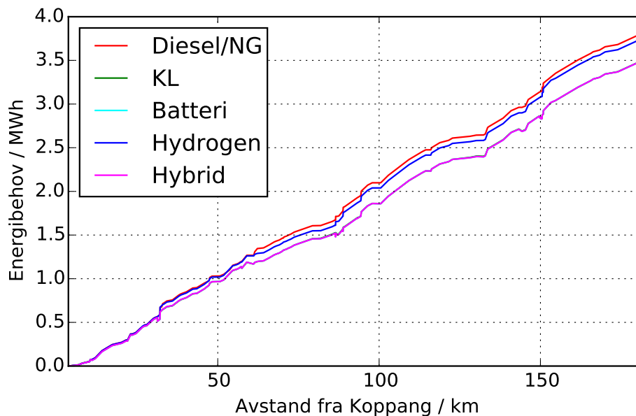
Figur 62: Energiforbruk for tømmertog fra Østerdalen (Koppang) over Rørros- og Solørbanen med forskjellige framdriftsteknologier.
