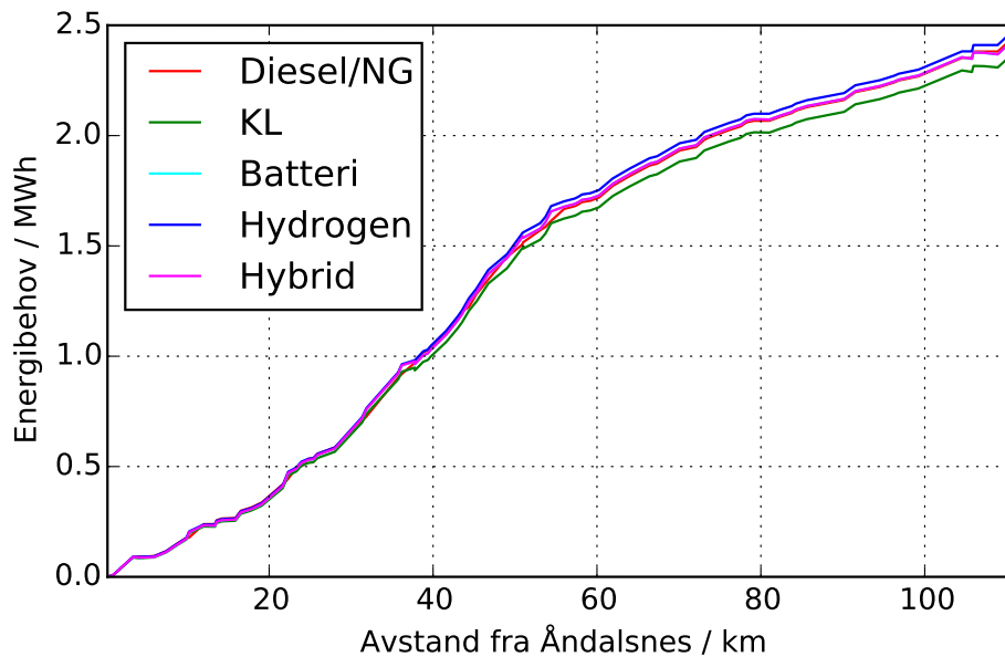
Figur 66: Energiforbruk for et godstog fra Åndalsnes til Dombås med forskjellige framdriftsteknologier.
