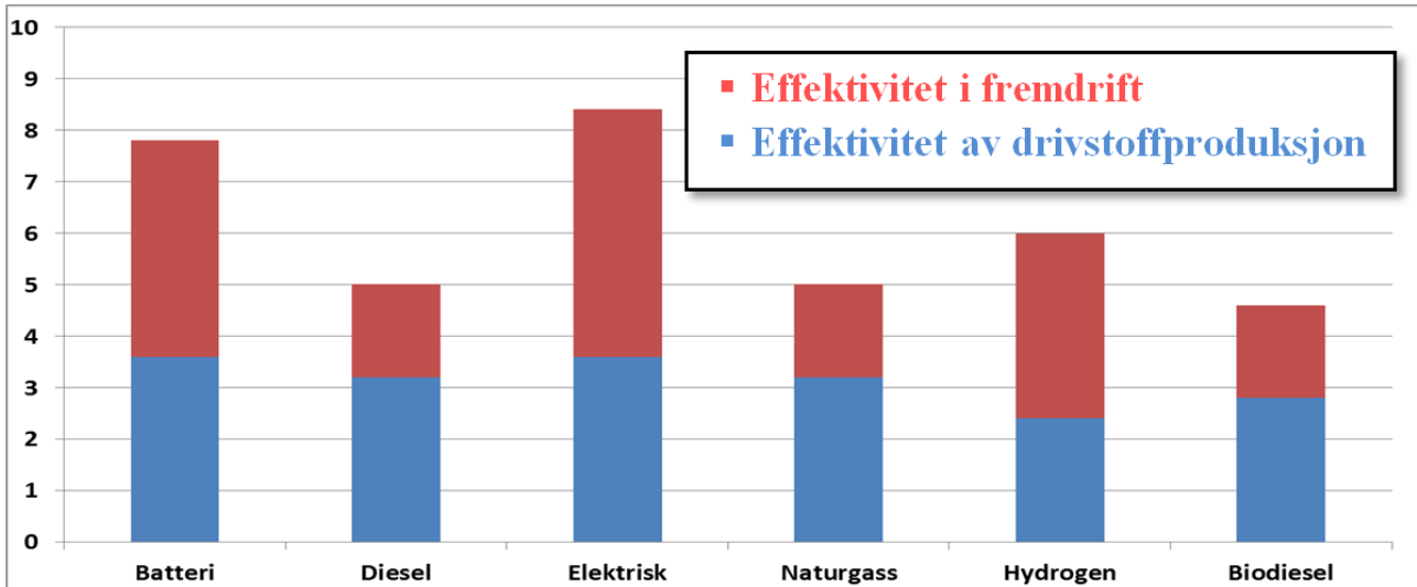
Figur 17: Resultater for energieffektivitet, underparameteren Effektivitet i fremdrift er vektet 60 %.
