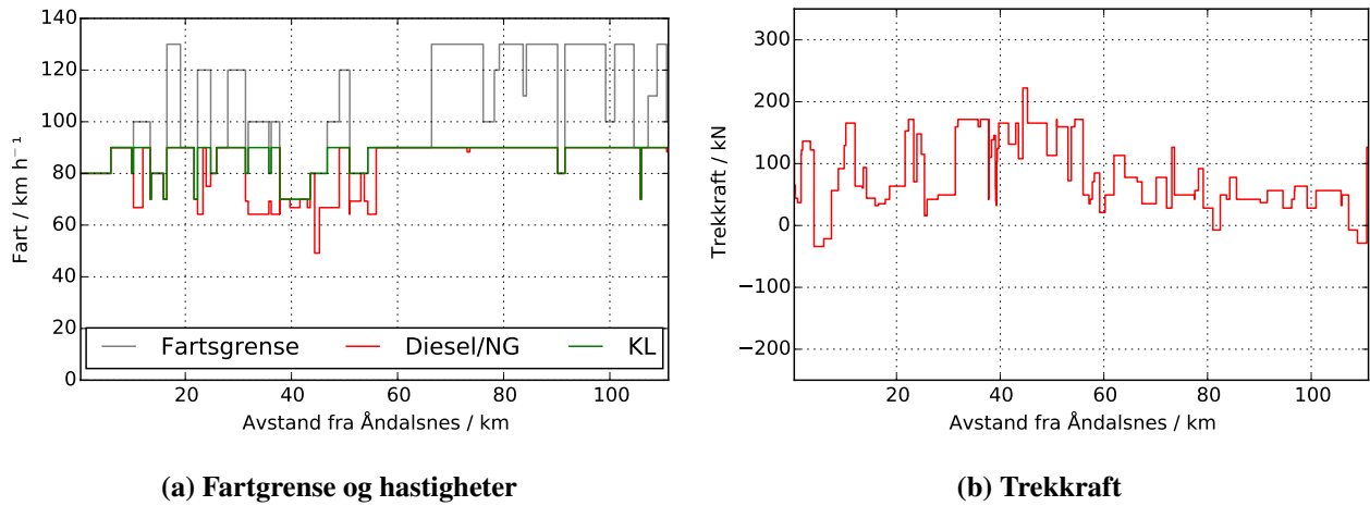
Figur 64: Nominelle hastigheter og trekkraft for et godstog (med halve lasten sammenlignet med referansegodstog) på vei fra Åndalsnes til Dombås. Hastighetene er noe forskjellige mellom diesel og elektrisk lokomotiv, mens trekkraften er omtrent det samme (diesel er plottet).
