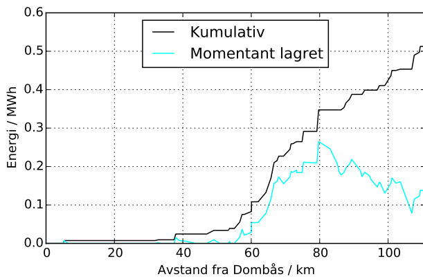
(a) Regenerativ bremsing
