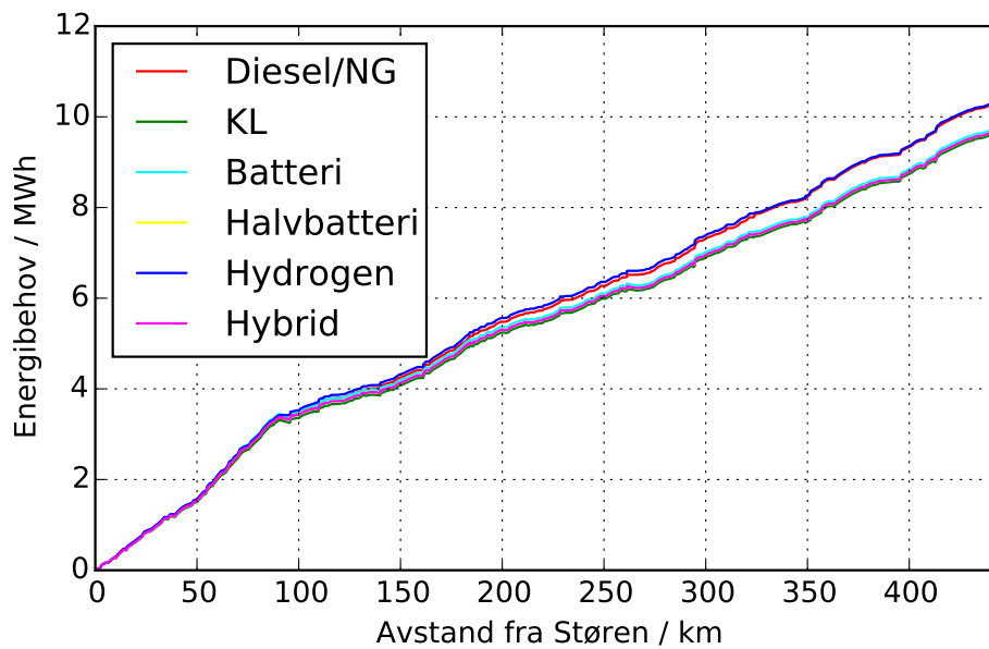
Figur 61: Energiforbruk for referansegodstoget over Rørros- og Solørbanen fra Støren til Kongsvinger med forskjellige framdriftsteknologier.
