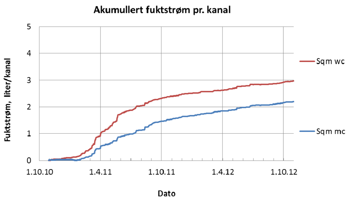
Figur 3.4 Diagram V5 (figur 3.4) viser samlet uttørking angitt i liter pr. luftkanal. Kurven merket Sqm wc gjelder fukt som er tørket ut med luftstrømmen gjennom vestre kanal og Sqm mc gjelder midtre kanal.
