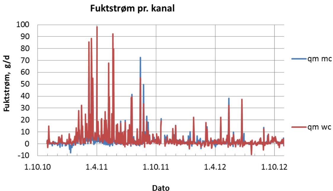
Figur 3.3 Diagram V9 (figur 3.3) viser beregnet fuktstrøm i de to instrumenterte kanalene. Fuktstrømmen er beregnet på grunnlag av luftstrømmen gjennom kanalen, vist i diagram V7 i Vedlegg, og forskjellen i absolutt fuktinnhold i luften ved de to kanalåpningene.
