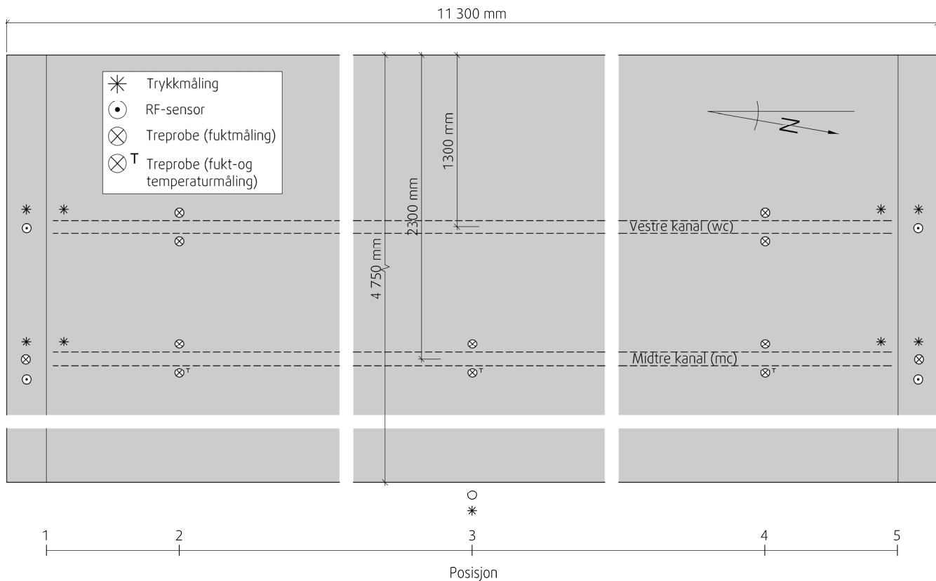
Figur 2.11 Planskisse over taket med både midtre kanal (mc) og vestre kanal (wc) med målesensorer for måling av trykk, RF, temperatur og trefuktighet.
