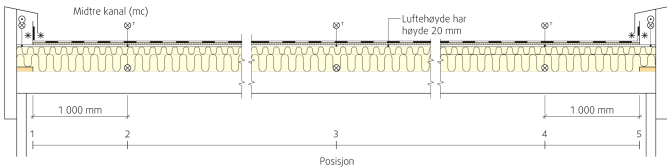
Fig 2.12 Snitt gjennom taket ved midtre kanal med plasseringen av sensorer både oppe i/ved luftkanalen og nede på dampsperra.
