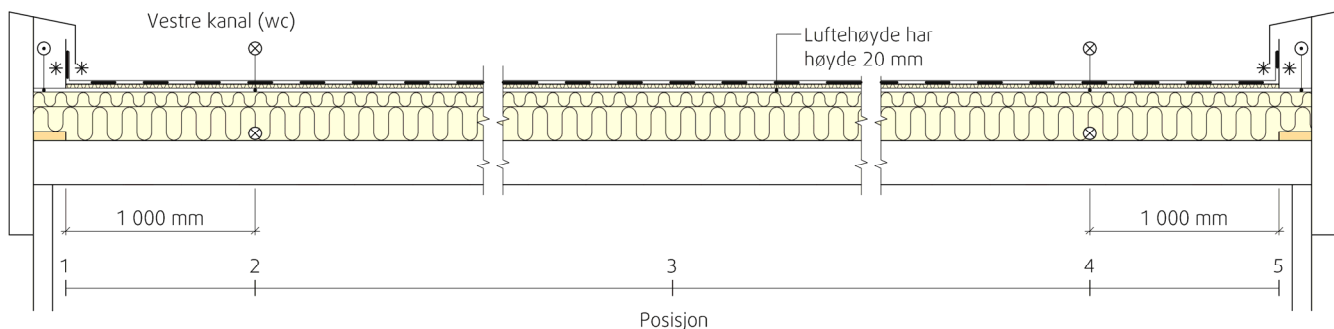
Fig 2.13 Snitt gjennom taket ved vestre kanal med plasseringen av sensorer både oppe i/ved luftkanalen og nede på dampsperra.
