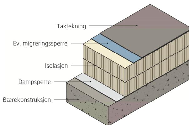
Figur 1.1 Tradisjonell oppbygning av rettvendt, kompakt tak uten lufting
